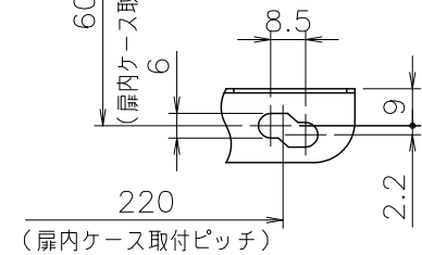
■イ部詳細図 (尺度1/2)
