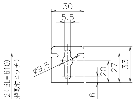
■A部詳細図 (尺度1/2)
