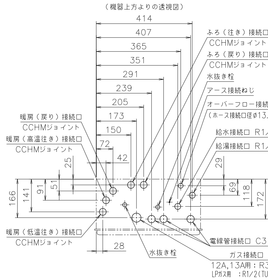
■底板よりの各継手高さ (mm)
