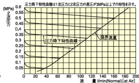
【GHSN-3 流量表】
