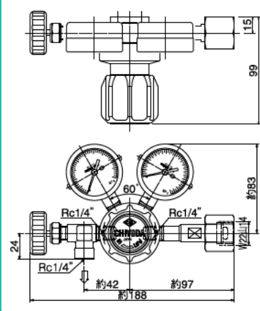
【外観寸法図】
