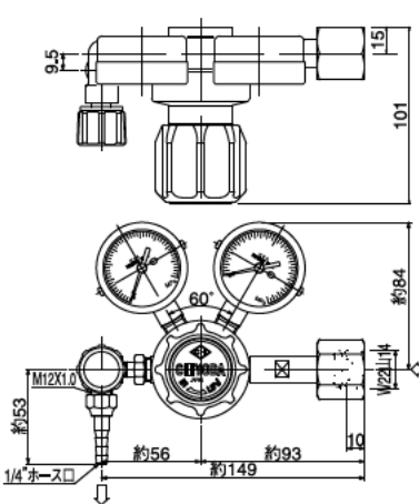
【外観寸法図】
