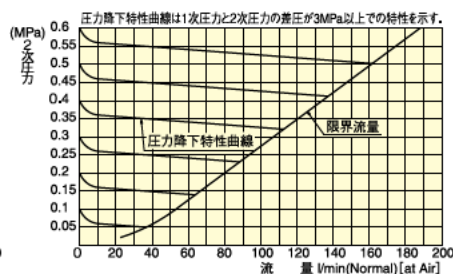
【GHSN-3 流量表】
