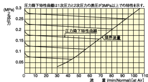
【GHN-3 流量表】
