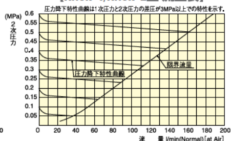
【AHSN-1/AHSN-2型 流量表】
