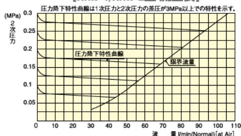
【AHN-1/AHSN-2型 流量表】
