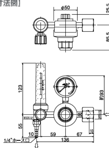
【外観寸法図】
