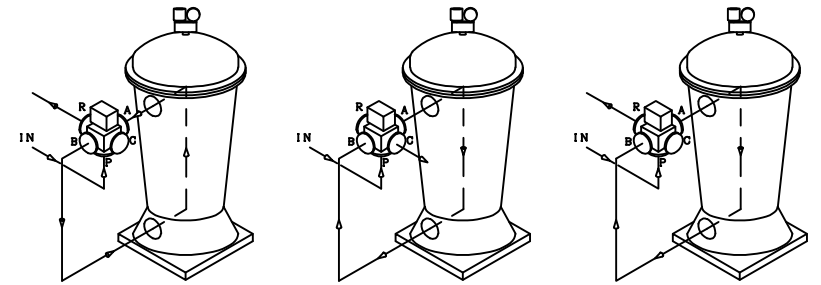
逆洗時流路
