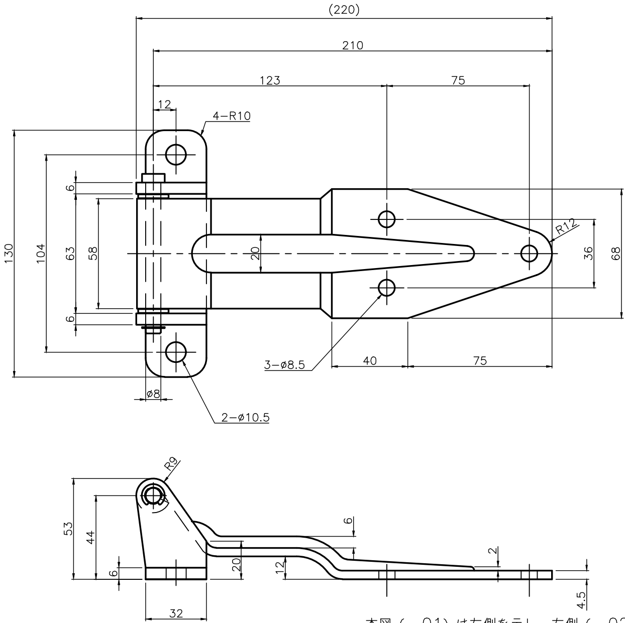
本図（－01）は左側を示し、右側（－02）は本図と対称とする。
