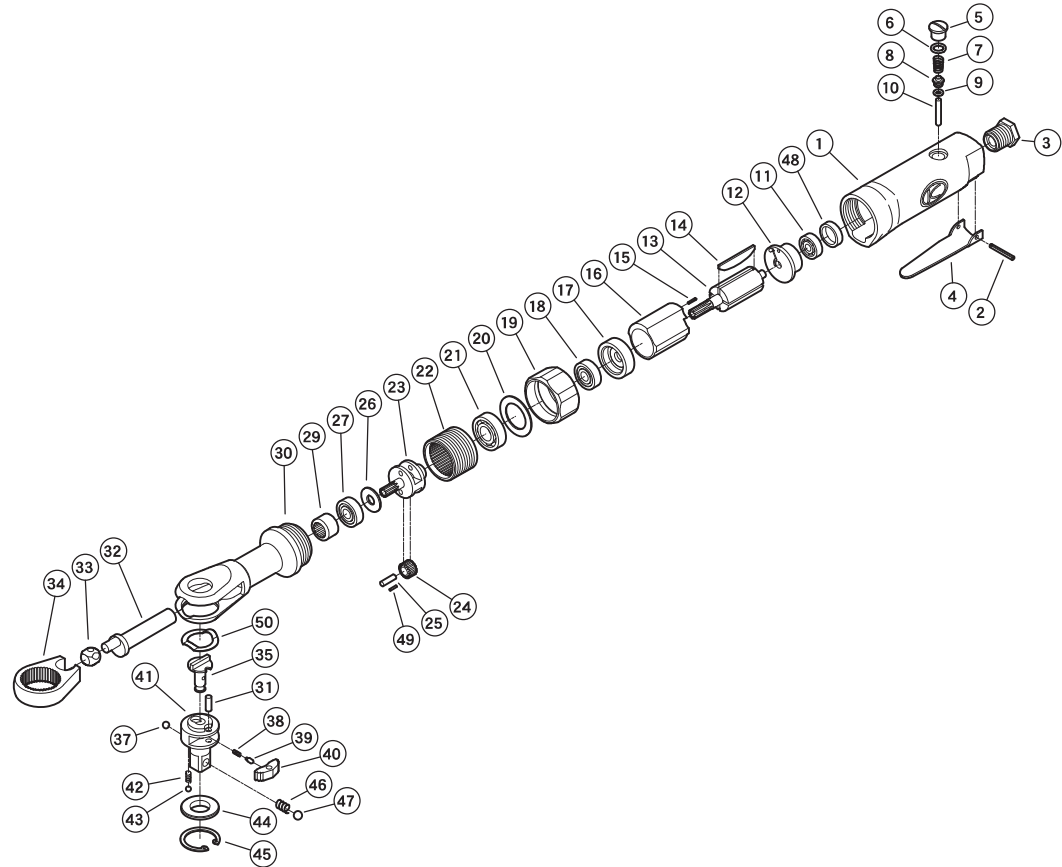
× ラチェットシャンクC.P構成パーツ
