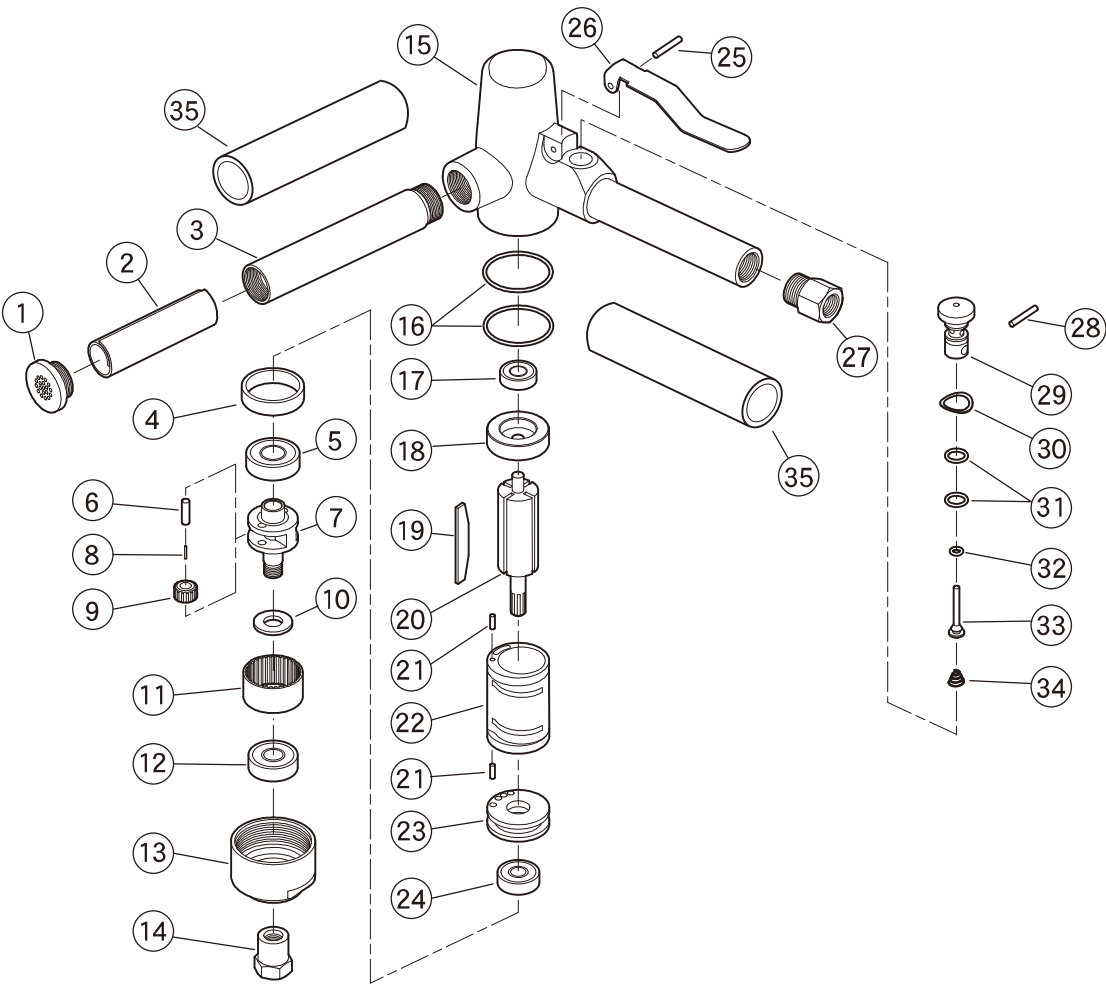
○ モータケースC.P構成パーツ
