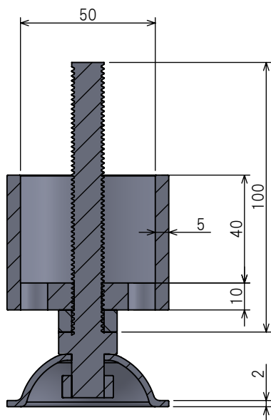
断面図 AU-AU
