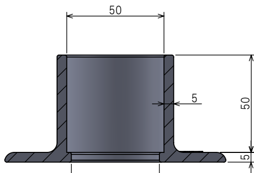
断面図 B-B
