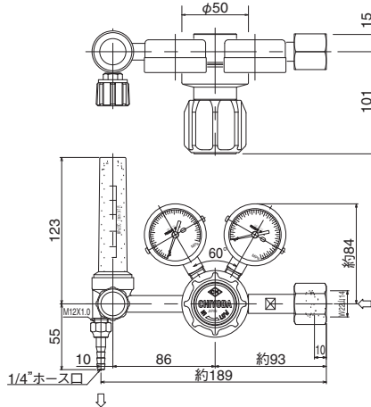
【外観寸法図】
