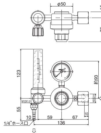
【外観寸法図】
