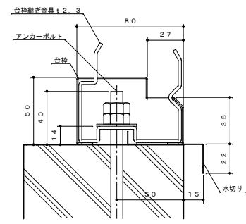
台枠、アンカー納まり詳細図 S=1:2
