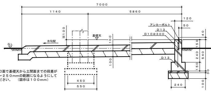
A-A断面図 S=1:20
