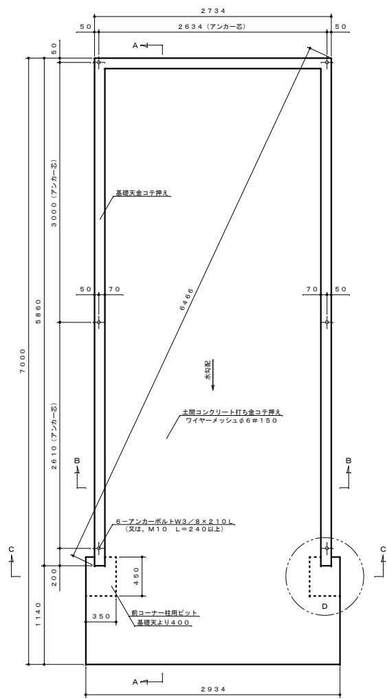
基礎伏せ図 S=1:30
