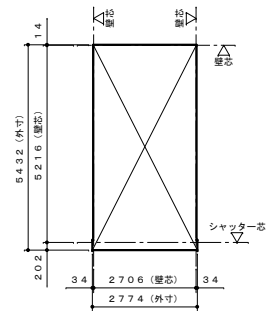
面積求積図 S=100
