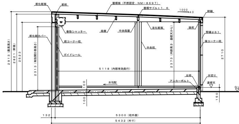
側面断面図 S=1:40
