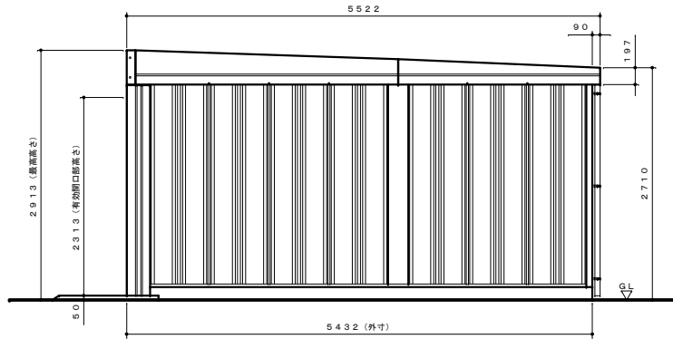
側面図 S=1:40
