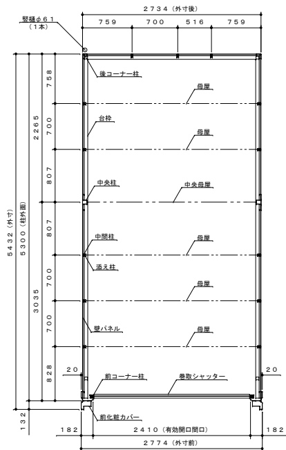
平面図 S=1:40
