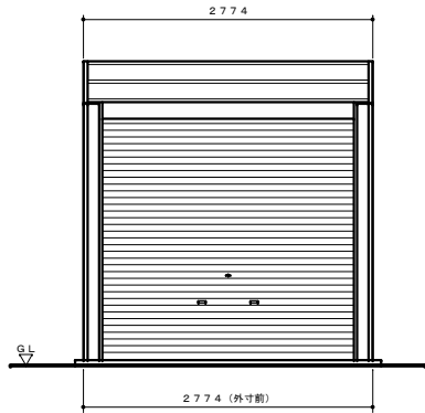
正面図 S=1:40
