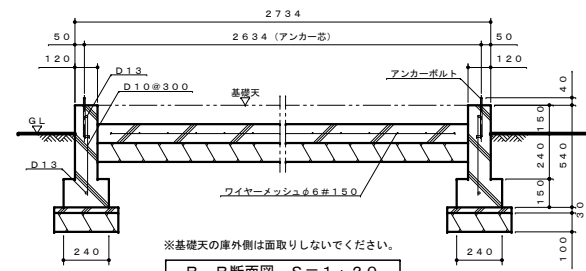
B-B断面図 S=1:20
