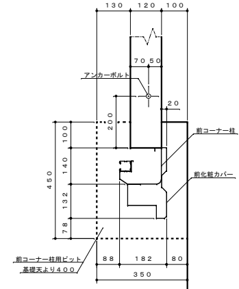
D部詳細図 S=1:10
