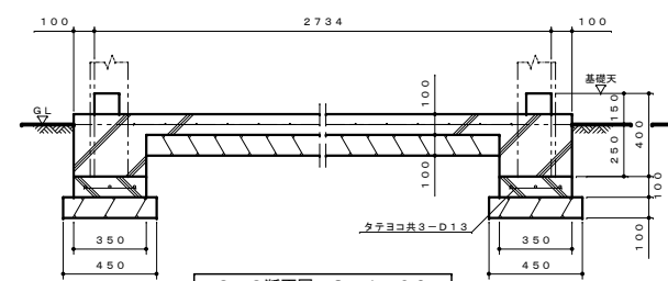
C-C断面図 S=1:20
