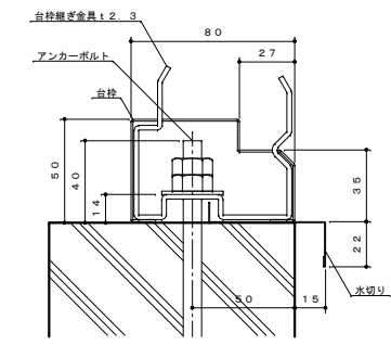
台枠、アンカー納まり詳細図 S=1:2 ※アンカーボルトの緩み止めに、ダブルナットで締め付けてください。
