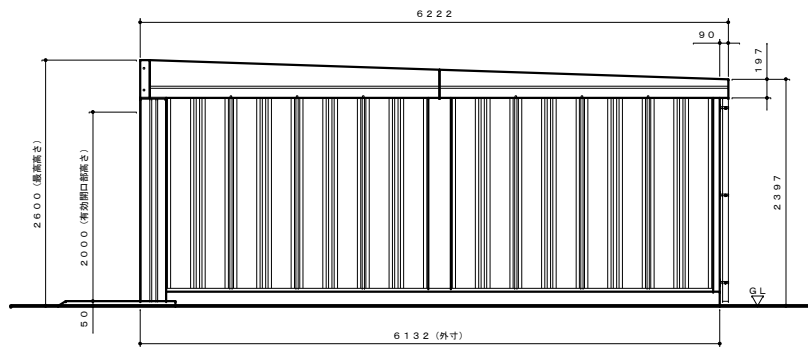
側面図 S=1:40
