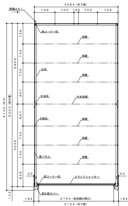
平面図 S=1:40
