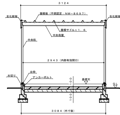
正面断面図 S=1:40
