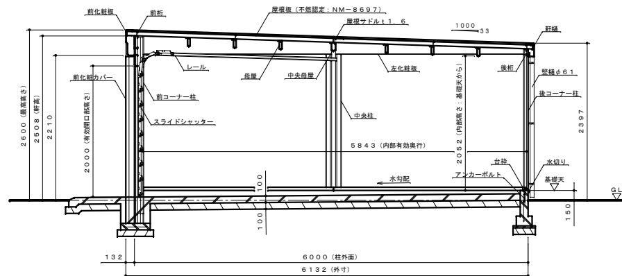
側面断面図 S=1:40
