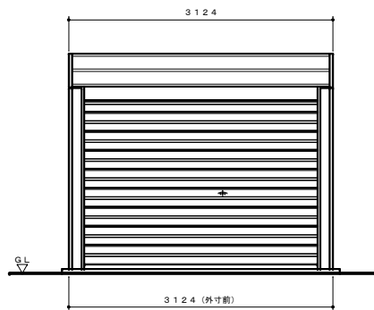
正面図 S=1:40
