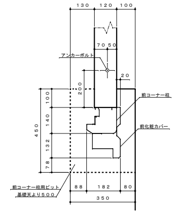
D部詳細図 S=1:10
