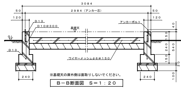
B-B断面図 S=1:20
