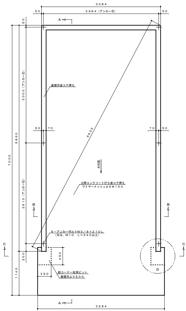
基礎伏せ図 S=1:30
