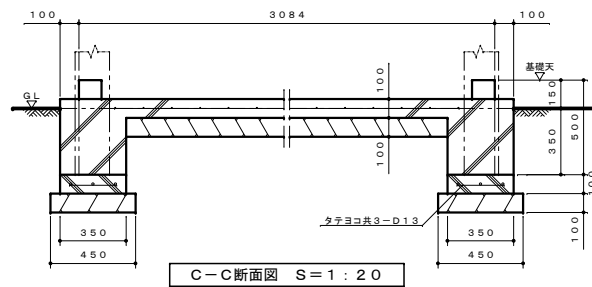
C-C断面図 S=1:20
