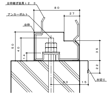
台枠、アンカー納まり詳細図 S=1:2
