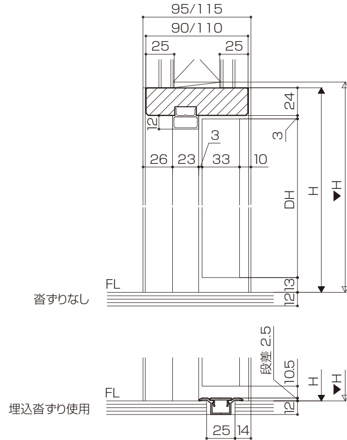
●縦断面図
