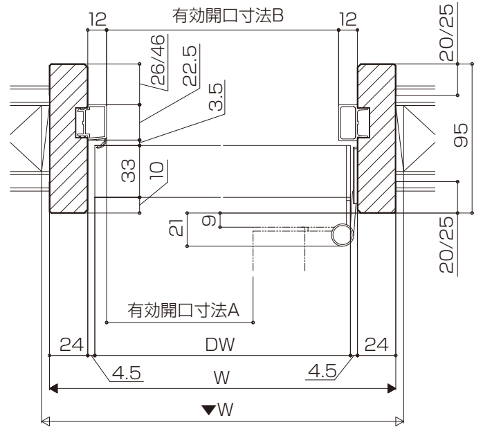
●横断面図
