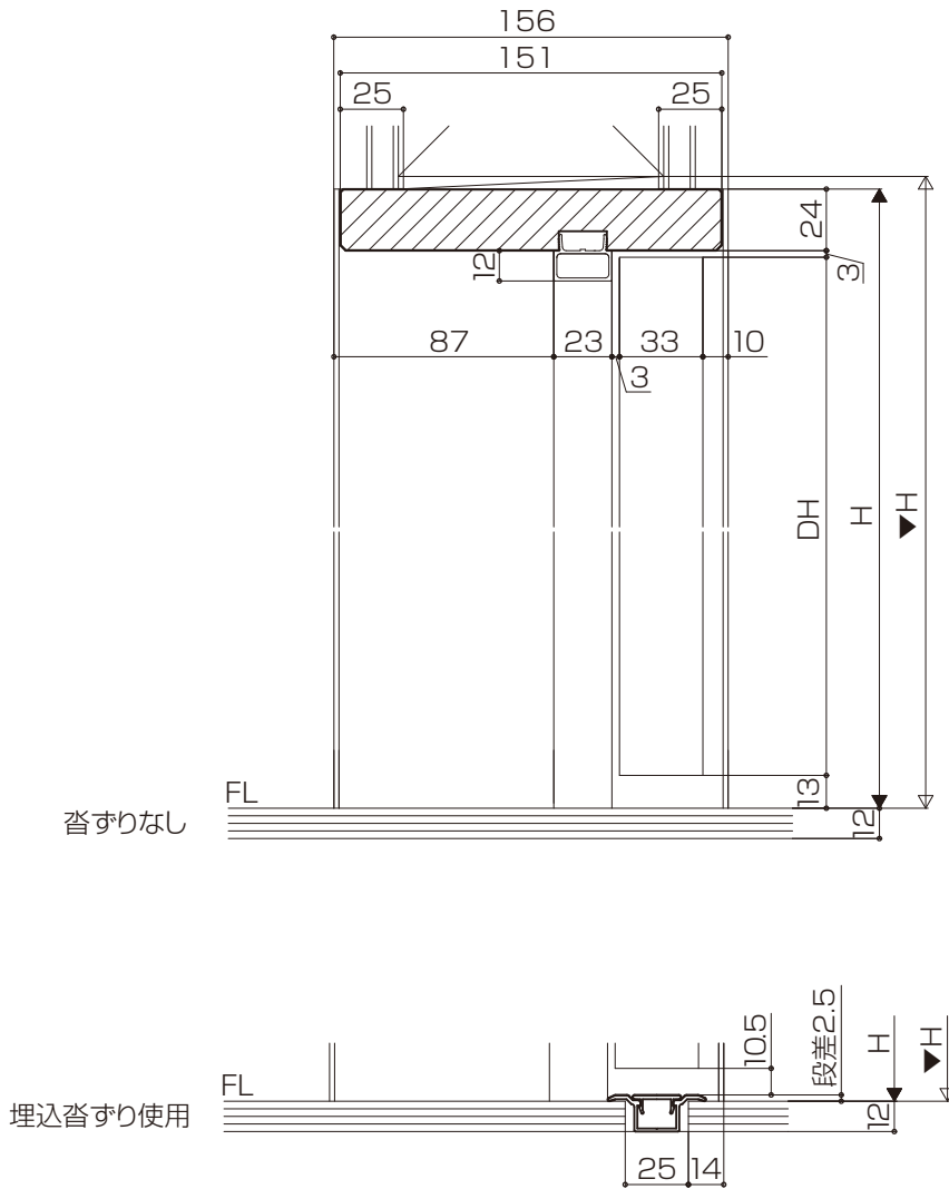
●縦断面図
