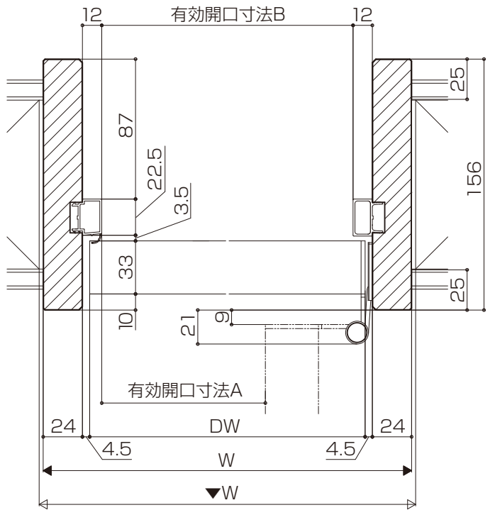
●横断面区
