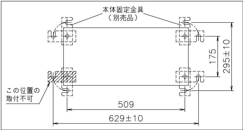
別売品の本体固定金具SETを使用する場合の基礎ボルト位置
