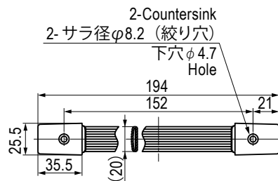
THA-318-1/THA-318B-1 (ツメなし) (Smooth Bottom)
