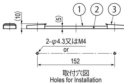
THA-318-1/THA-318B-1 (ツメなし) (Smooth Bottom)
