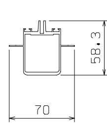
⑤ 中間梁
