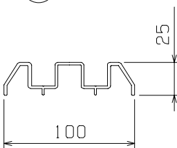
⑪ 下レール
