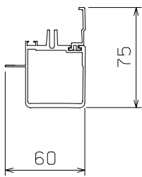
④ 正面梁
