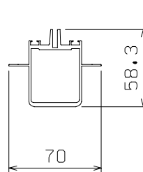
⑤ 中間梁
