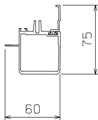
④ 正面梁
