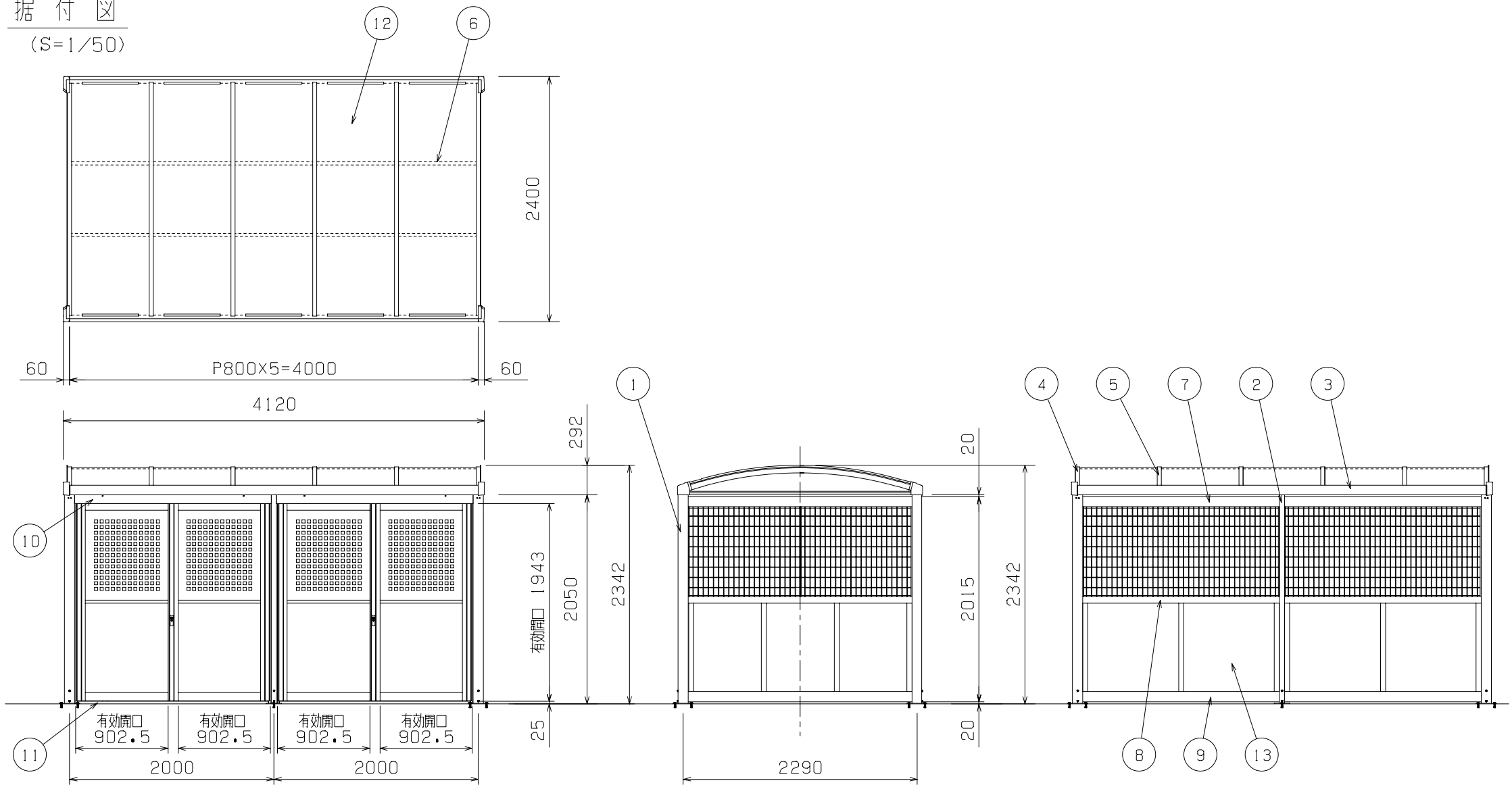
④ 正面梁
