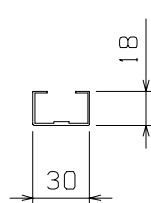
⑥ 母屋
