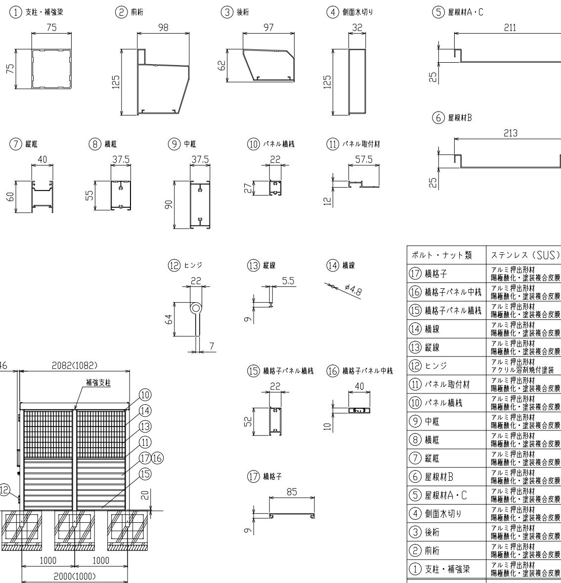
主要部材断面 (S=1/5)
