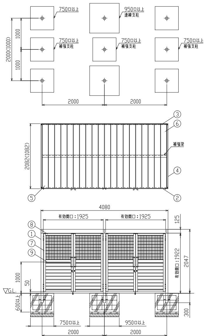
据 付 図 (S=1/50)
