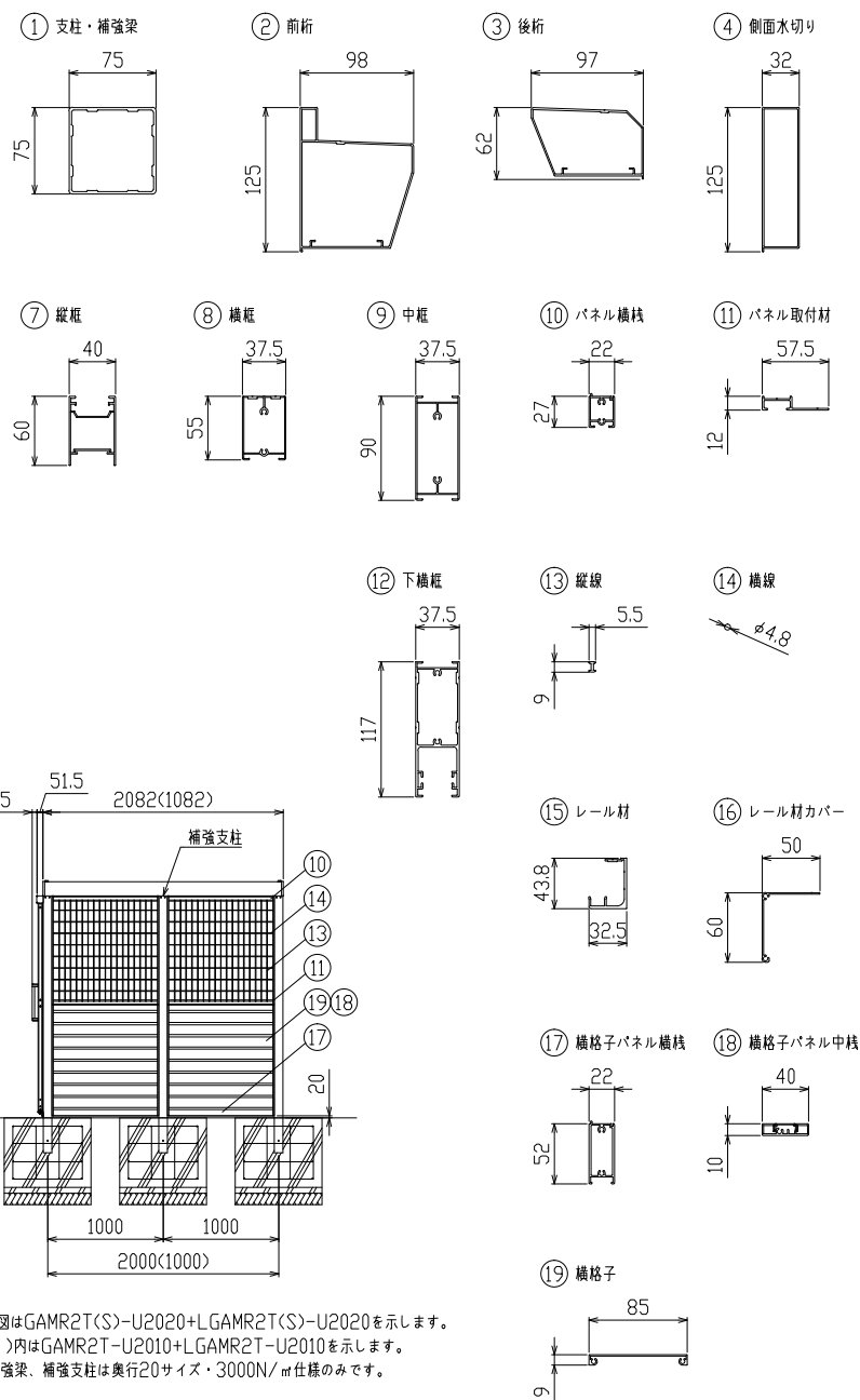
主要部材断面 (S=1/5)
