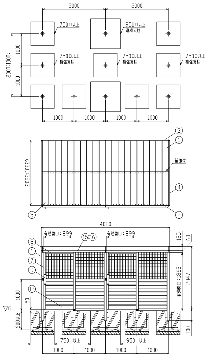
据付図 (S=1/50)
