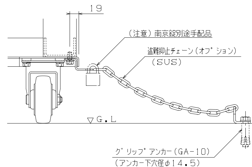
盗難抑止チェーン取付部詳細 (S = 1 / 5)
