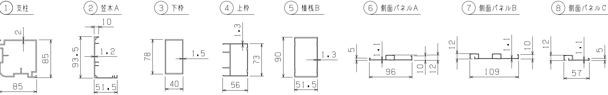
主要部材断面図 (S=1/5)
