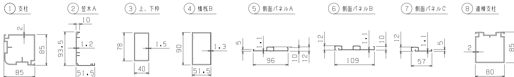
主要部材断面図 (S=1/5)
