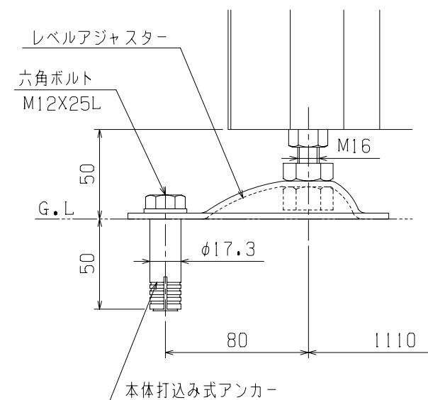
B部詳細図 (S=1/3)
