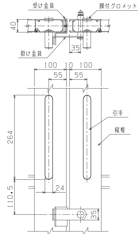
A部詳細図 (S=1/6)
