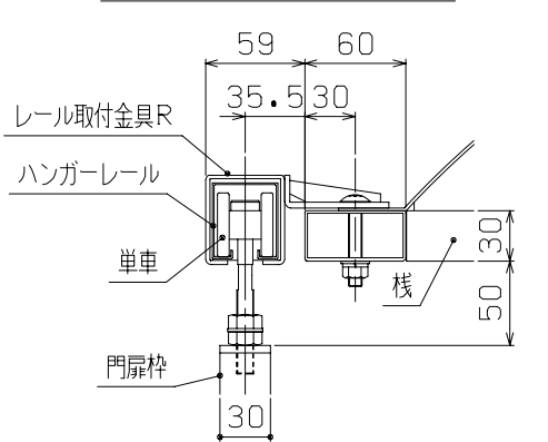
E-E断面図 (1/5)
