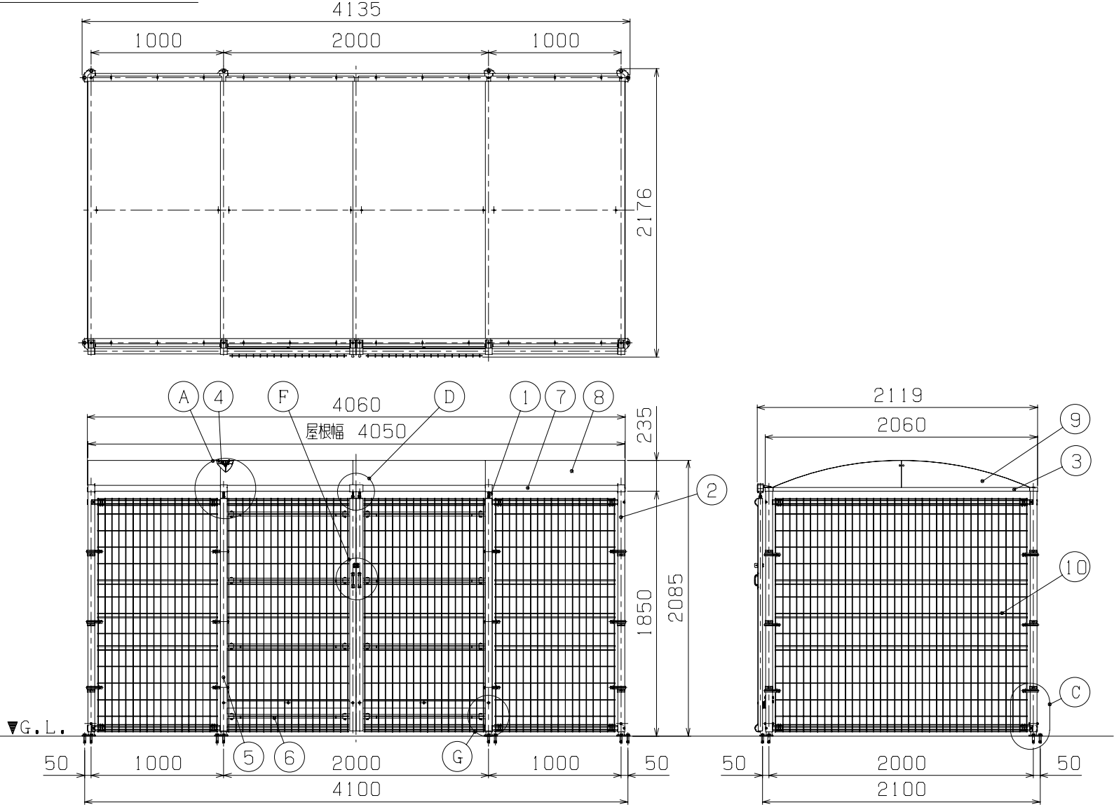
据付図 (1/40)
