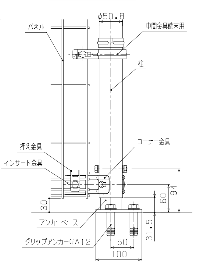
C部詳細図 (1/5)
