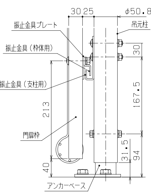
G部側面詳細図 (1/5)
