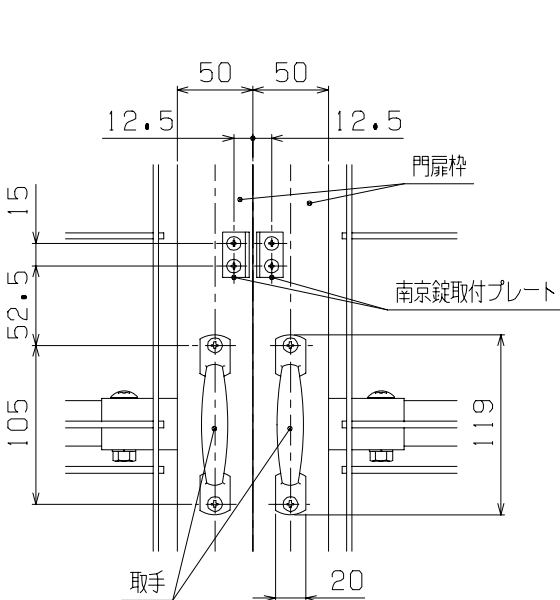
F部詳細図 (1/5)
