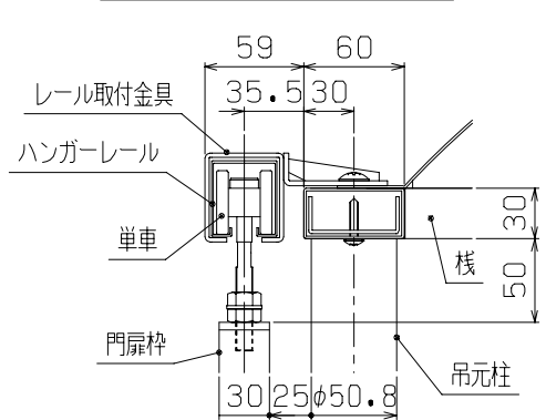
B-B断面図 (1/5)
