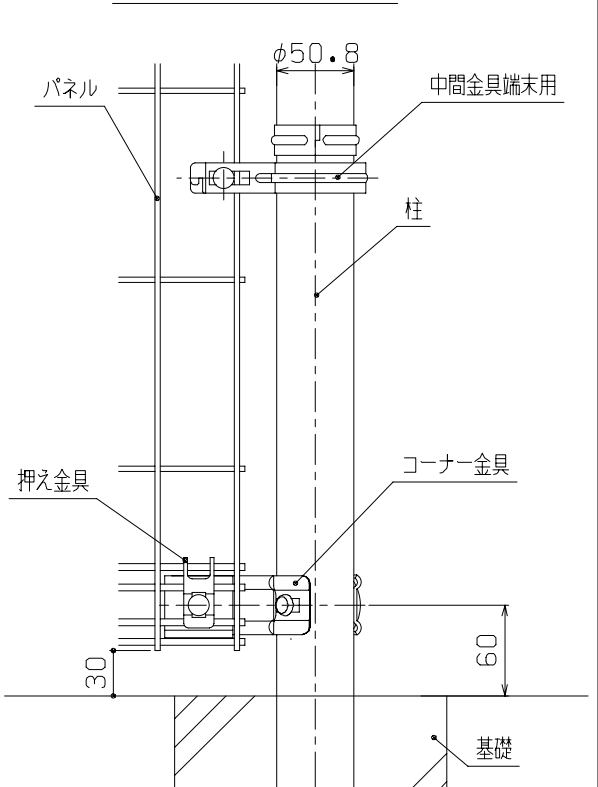
C部詳細図 (1/5)
