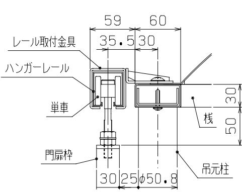
B-B断面図 (1/5)
