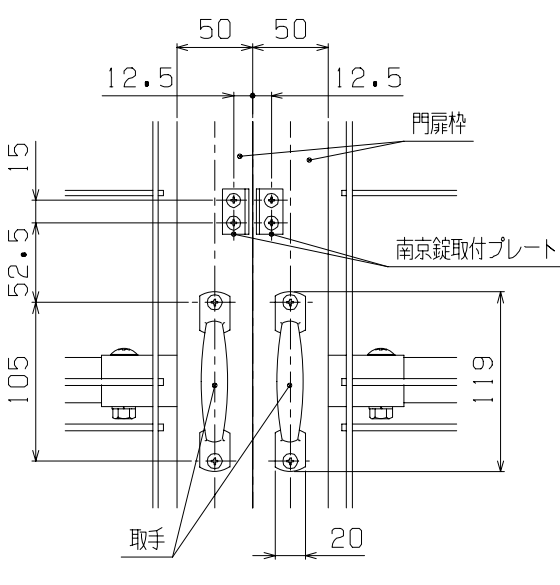
F部詳細図 (1/5)
