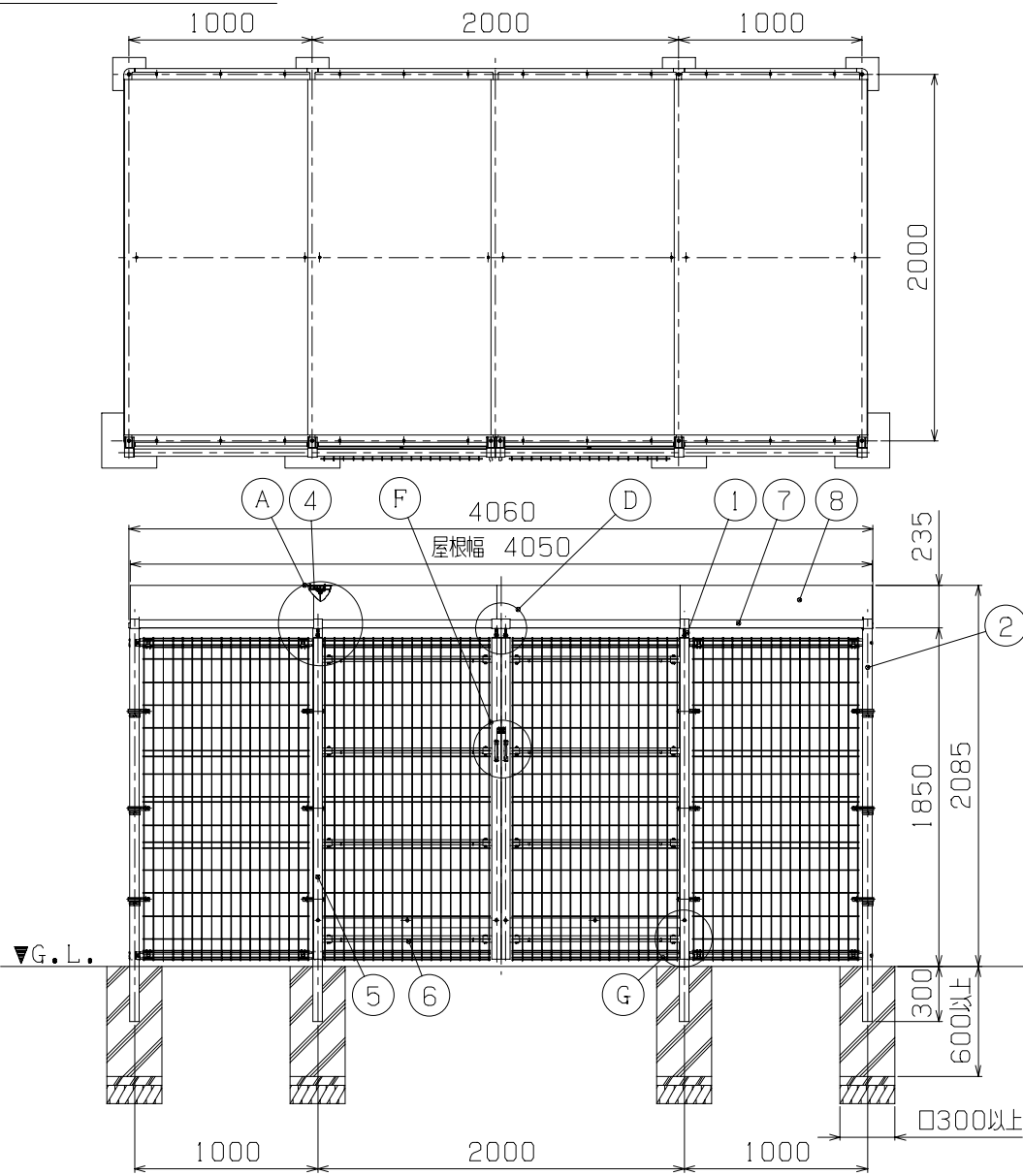
据付図 (1/40)
