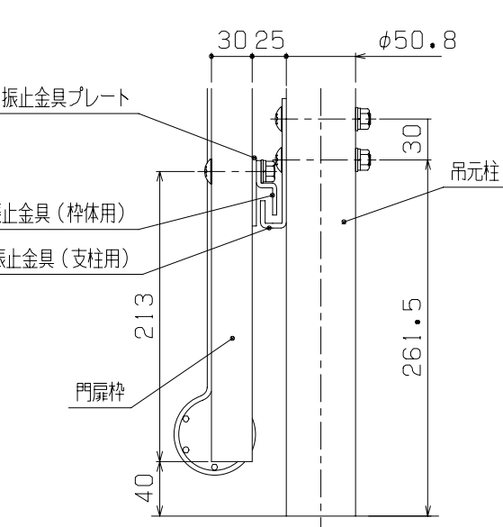
G部側面詳細図 (1/5)
