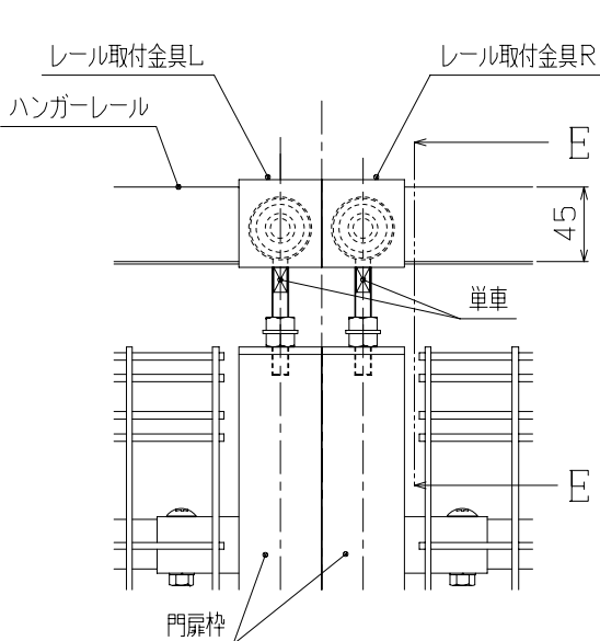
D部詳細図 (1/5)
