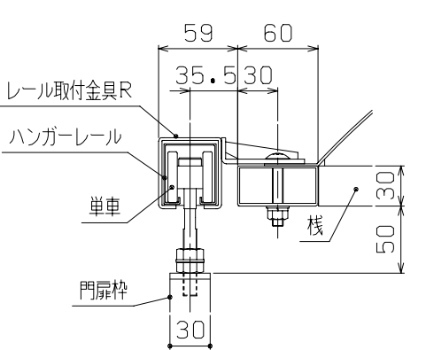
E-E断面図 (1/5)
