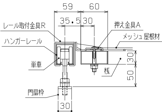
E-E断面図 (1/5)
