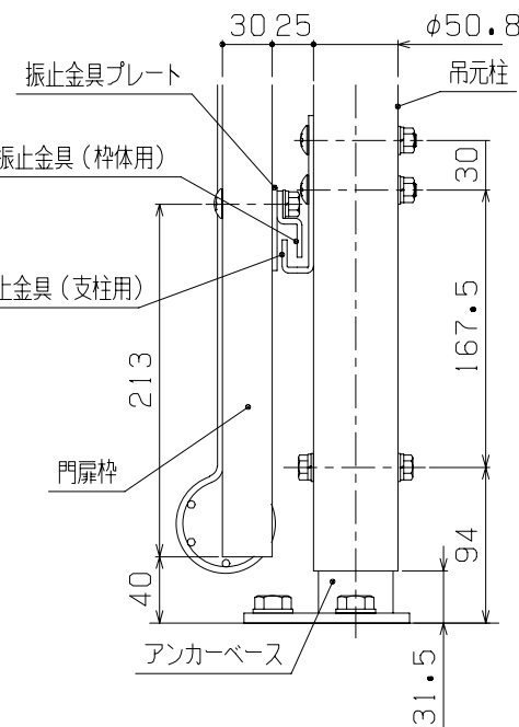
G部側面詳細図 (1/5)
