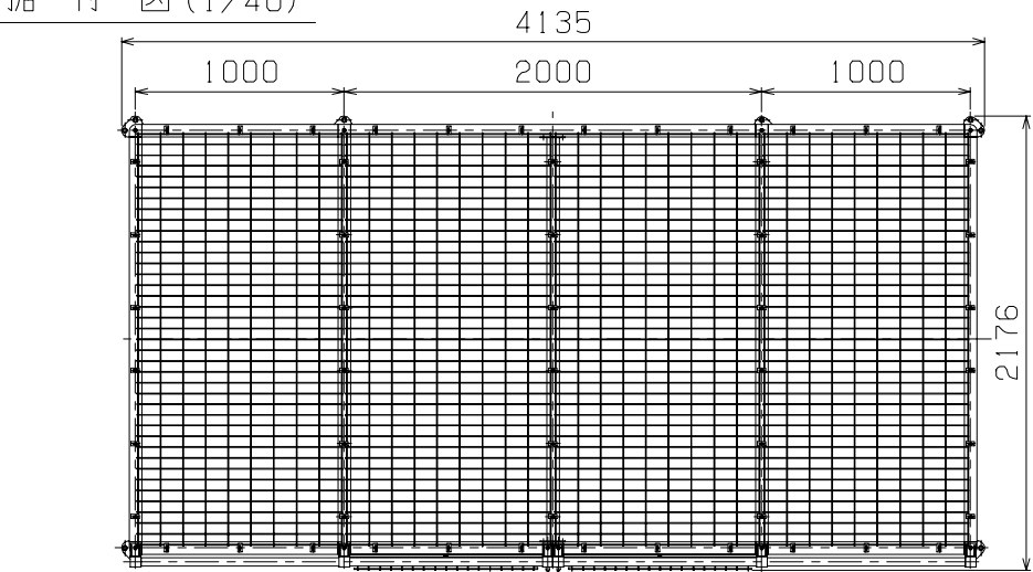
据付図 (1/40)
