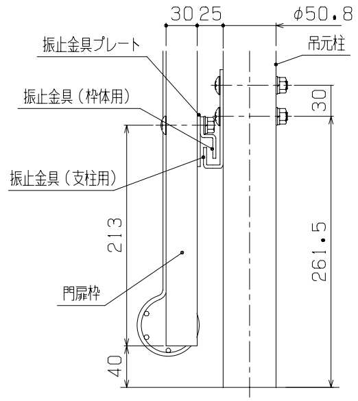
G部側面詳細図 (1/5)
