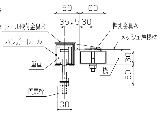
E-E断面図 (1/5)
