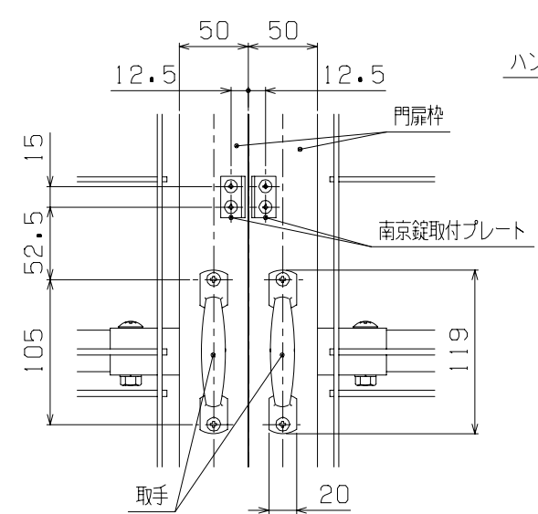
F部詳細図 (1/5)
