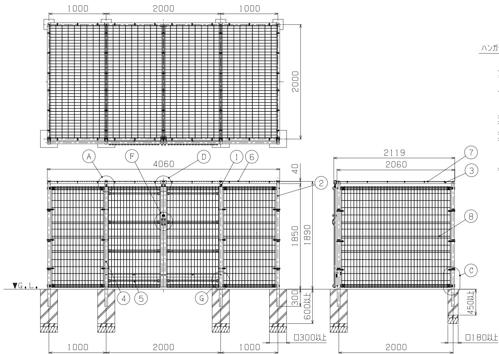
据付図 (1/40)
