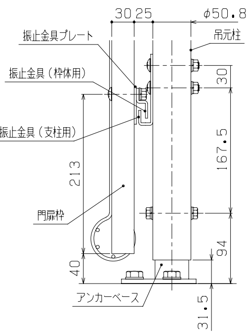
G部側面詳細図 (1/5)
