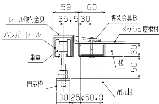
E-E断面図 (1/5)
