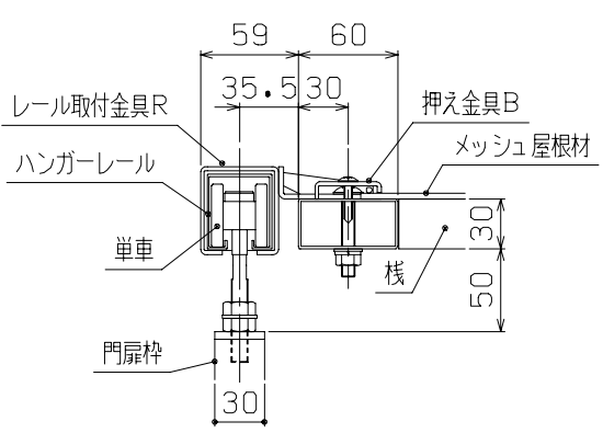
E-E断面図 (1/5)
