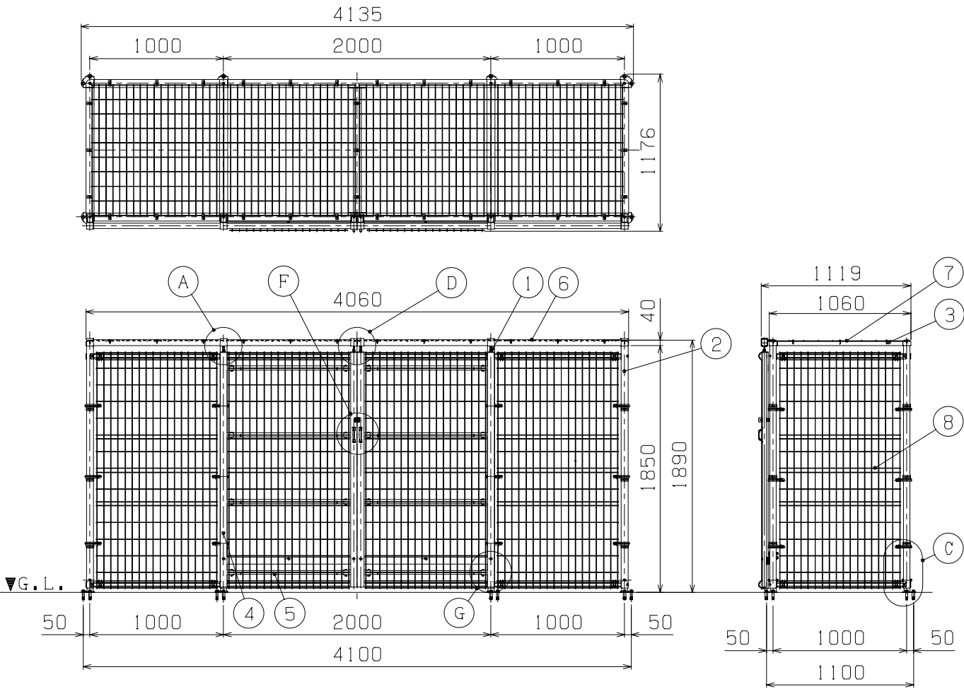
据付図 (1/40)
