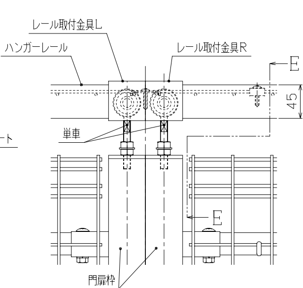
D部詳細図 (1/5)
