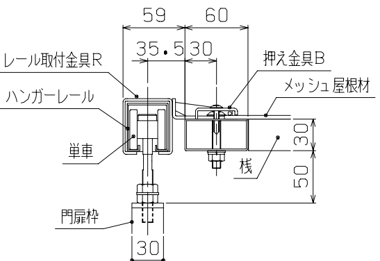
E-E断面図 (1/5)
