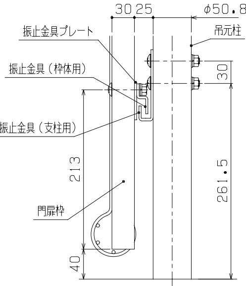
G部側面詳細図 (1/5)
