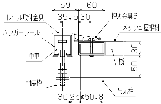
E-E断面図 (1/5)
