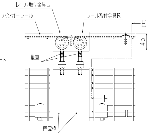
D部詳細図 (1/5)
