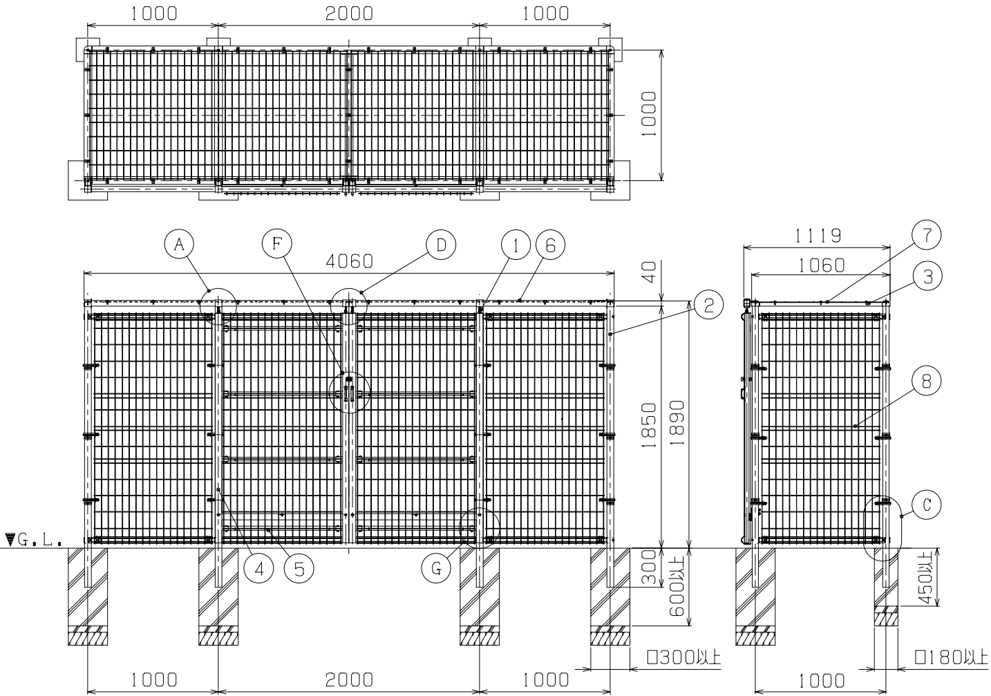
据付図 (1/40)
