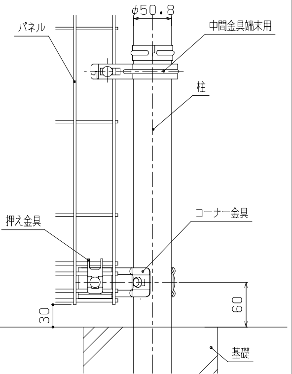
C部詳細図 (1/5)
