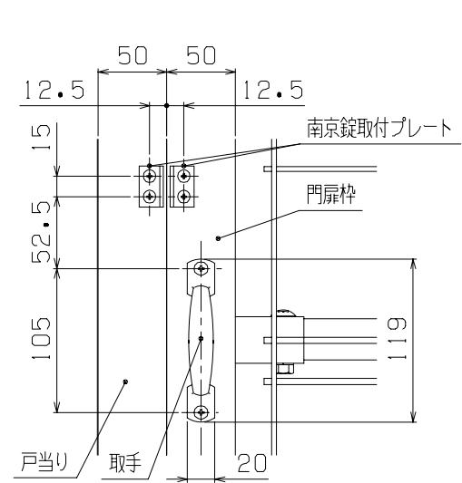
D部詳細図 (1/5)
