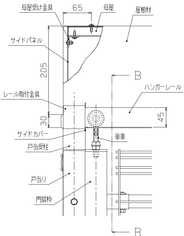
A部詳細図 (1/5)
