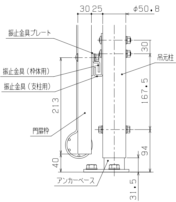
E部側面詳細図 (1/5)
