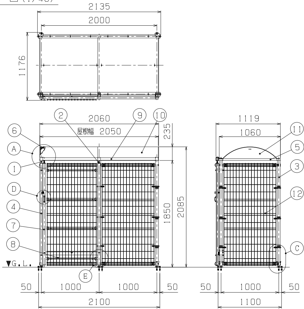
据付図 (1/40)
