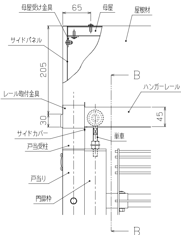
A部詳細図 (1/5)
