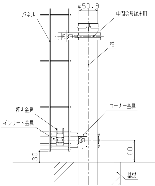
C部詳細図 (1/5)
