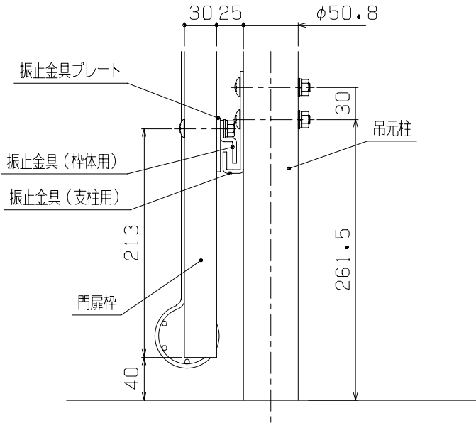
E部側面詳細図 (1/5)
