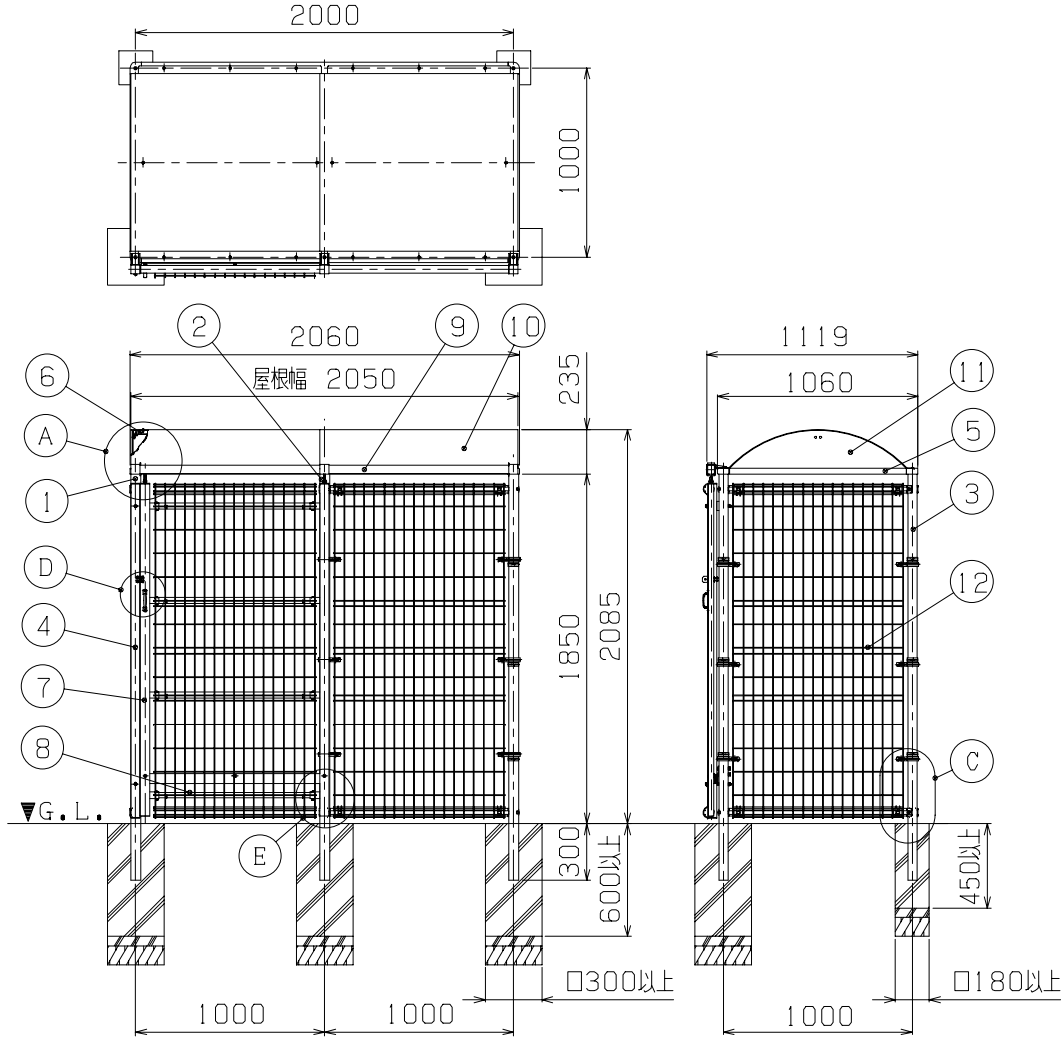
据付図 (1/40)
