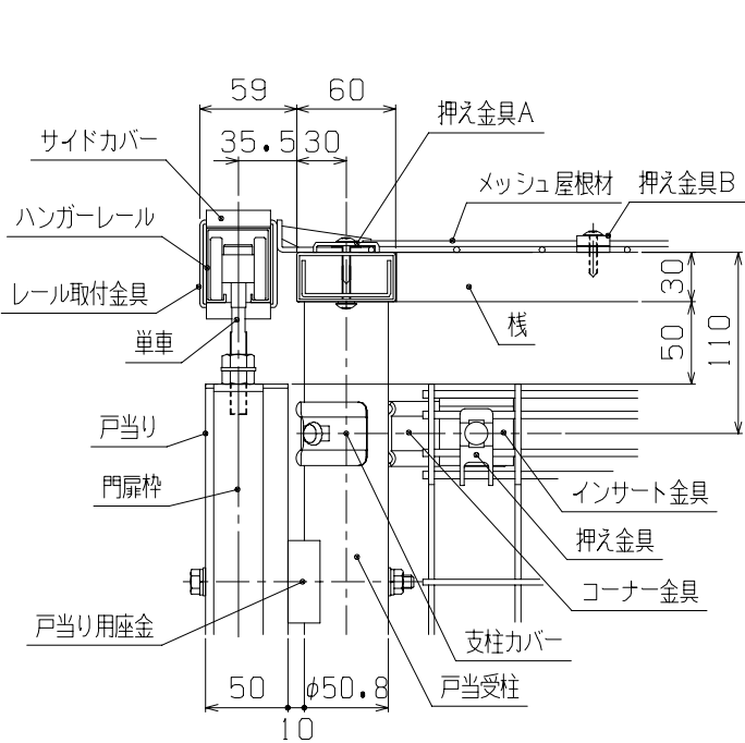
B-B断面図 (1/5)
