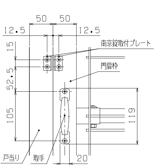
D部詳細図 (1/5)
