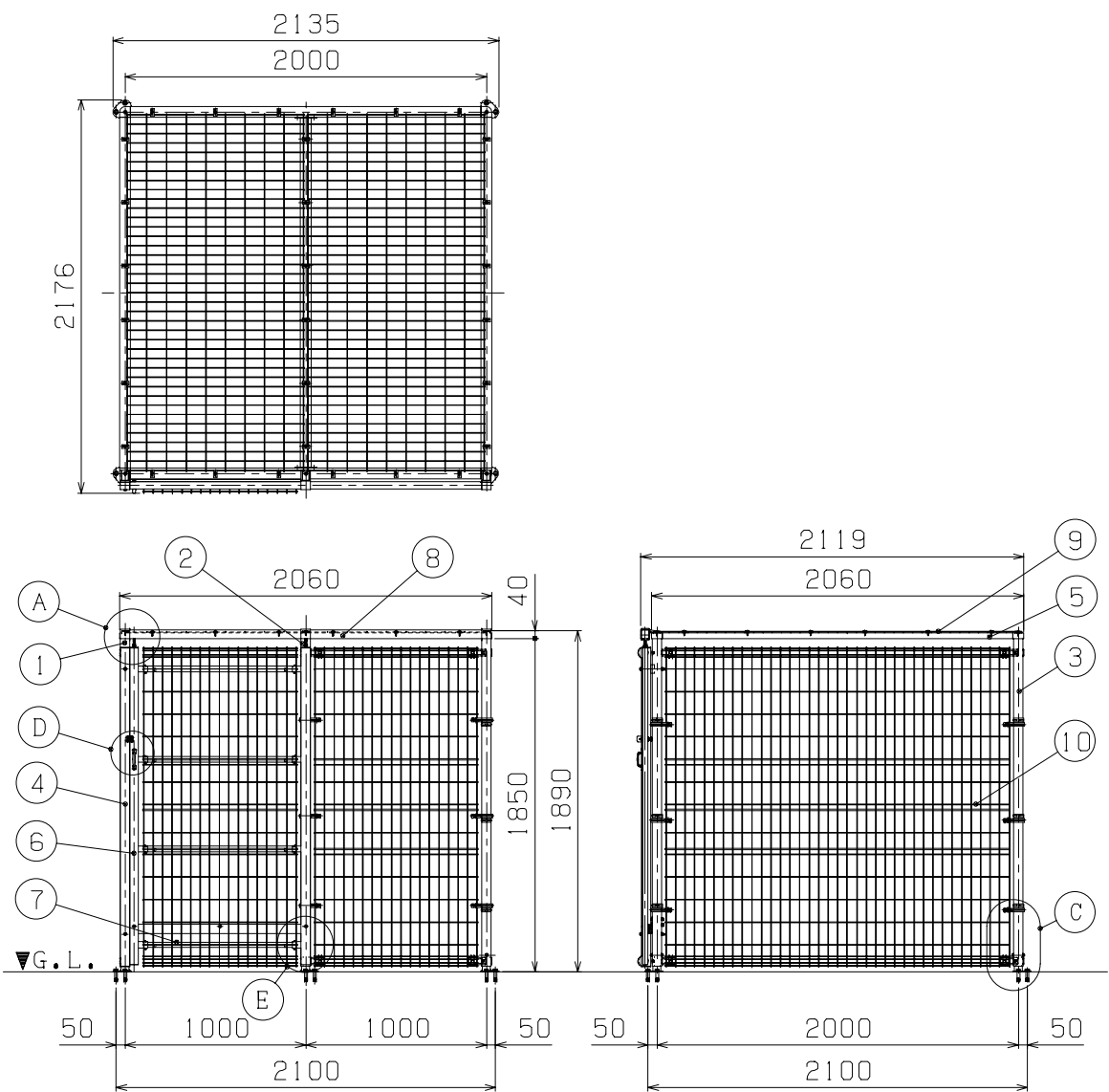
据付図 (1/40)
