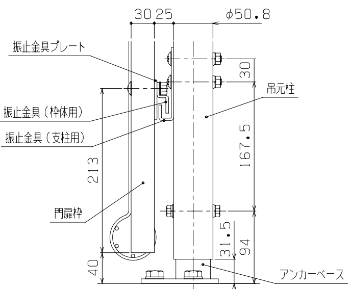
E部側面詳細図 (1/5)
