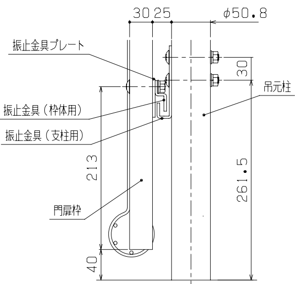
E部側面詳細図 (1/5)
