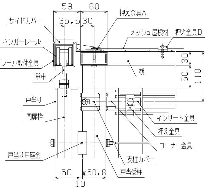
B-B断面図 (1/5)
