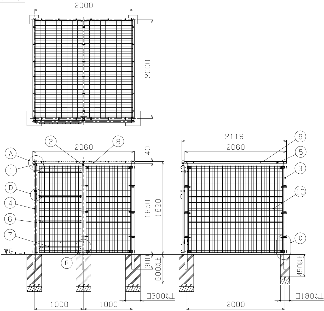
据付図 (1/40)
