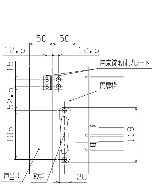
D部詳細図 (1/5)
