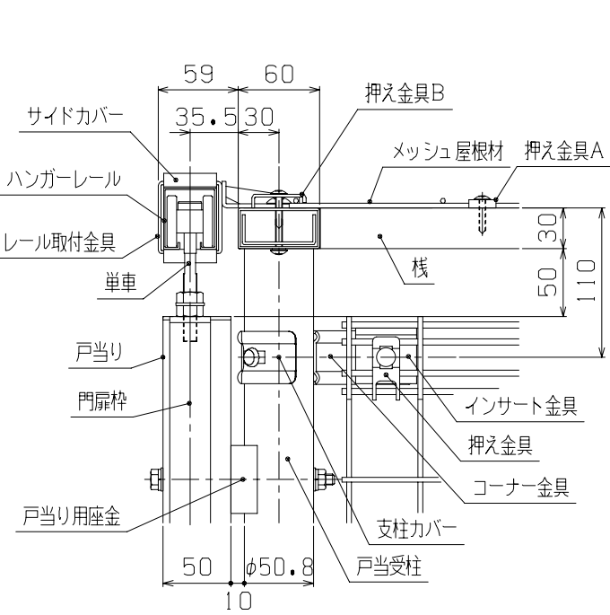
B-B断面図 (1/5)
