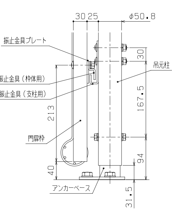
E部側面詳細図 (1/5)
