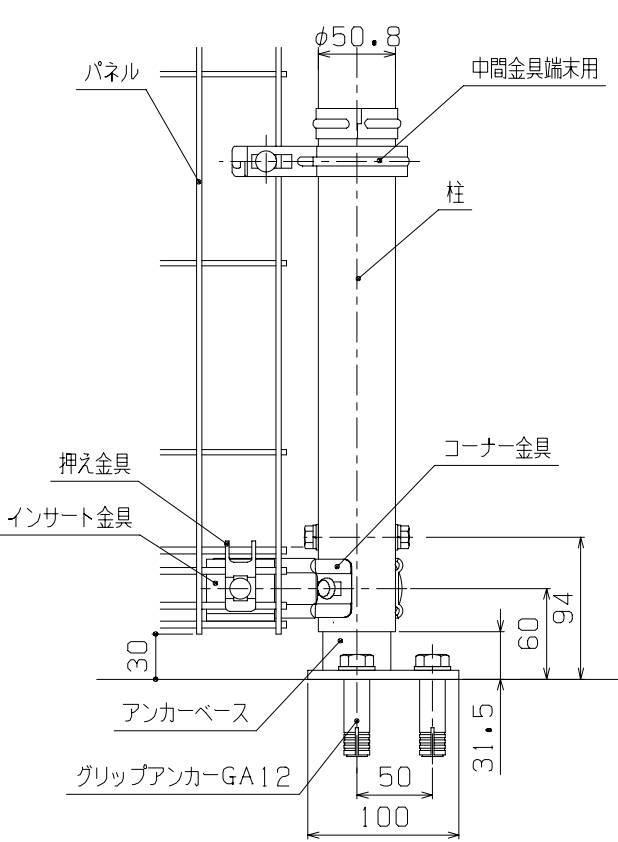
C部詳細図 (1/5)
