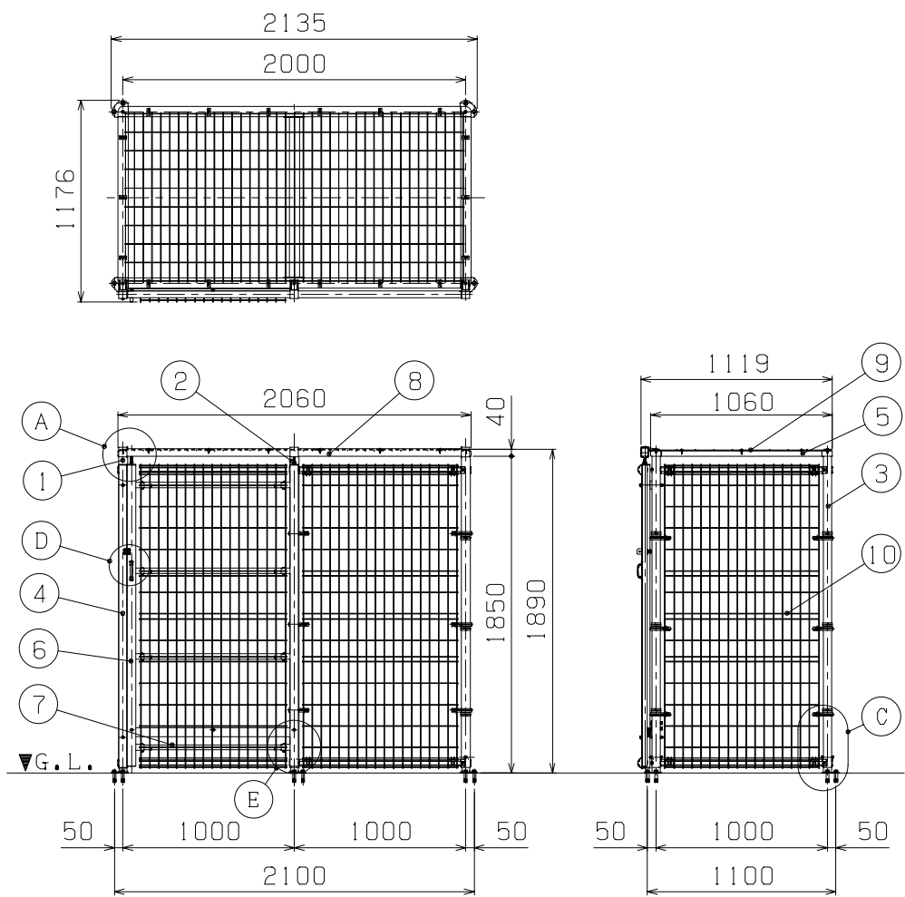
据付図 (1/40)
