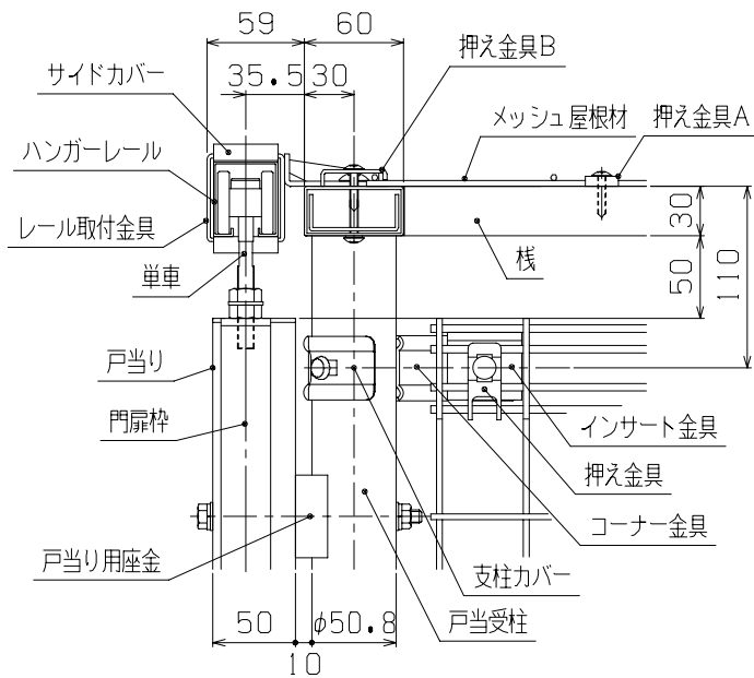
B-B断面図 (1/5)
