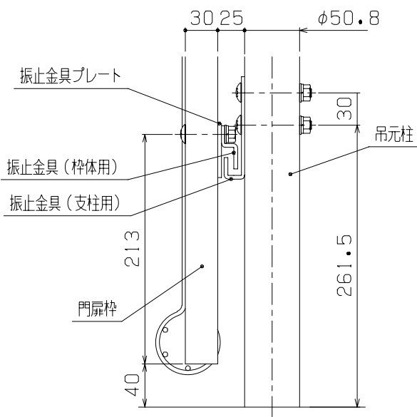
E 部側面詳細図 (1/5)
