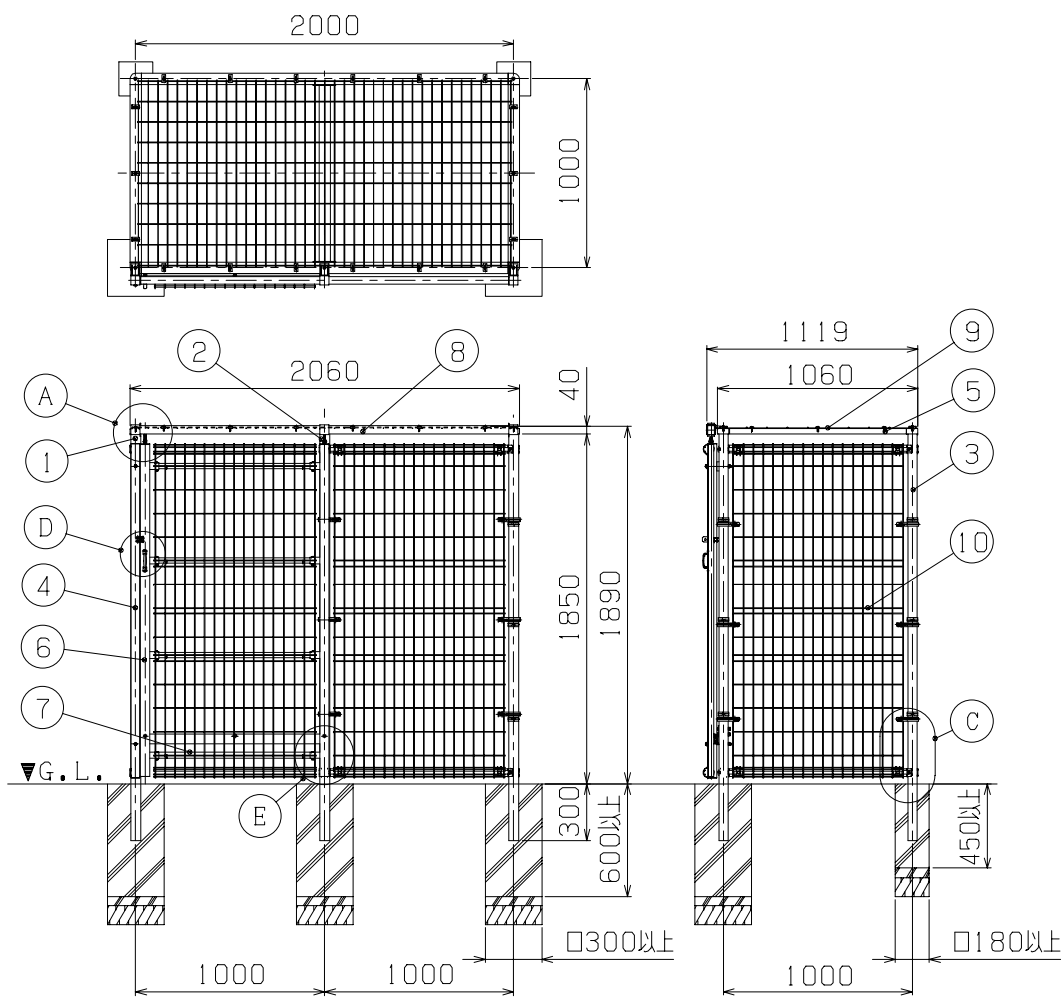
据 付 図 (1/40)
