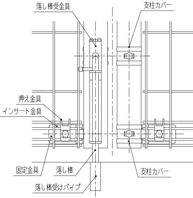
D部詳細図 (1/5)
