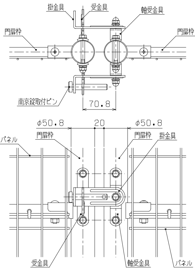
A部詳細図 (1/5)
