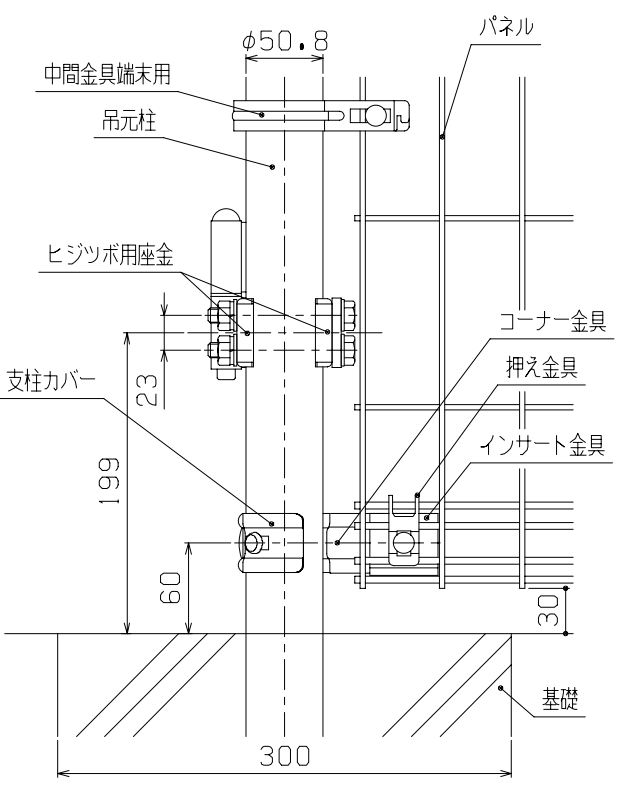
B部詳細図 (1/5)
