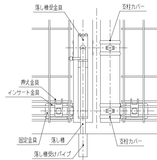
D 部詳細図 (1/5)
