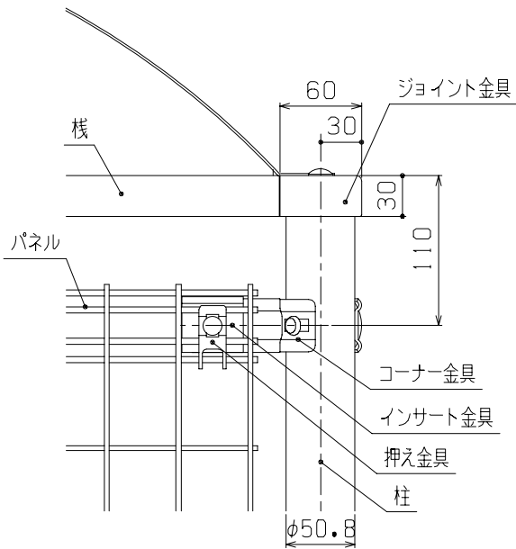
C部詳細図 (1/5)
