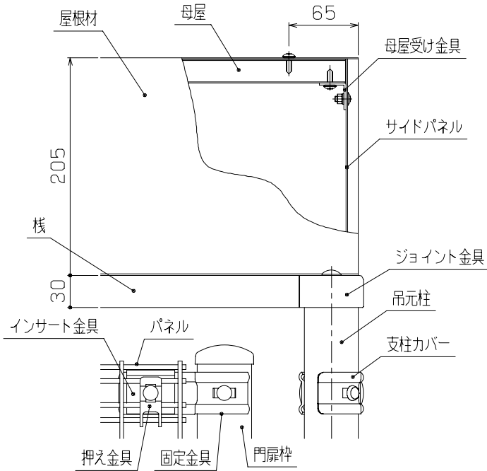
D部詳細図 (1/5)
