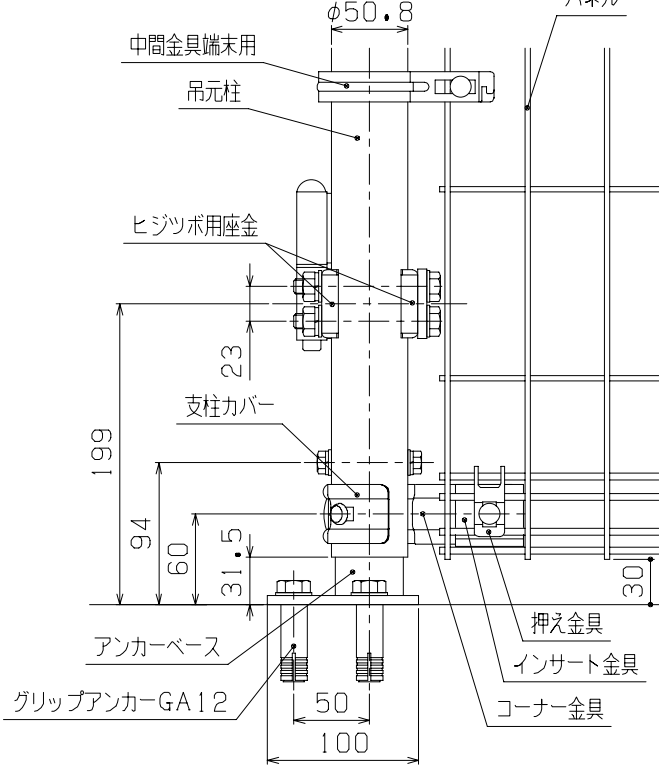
B部詳細図 (1/5)
