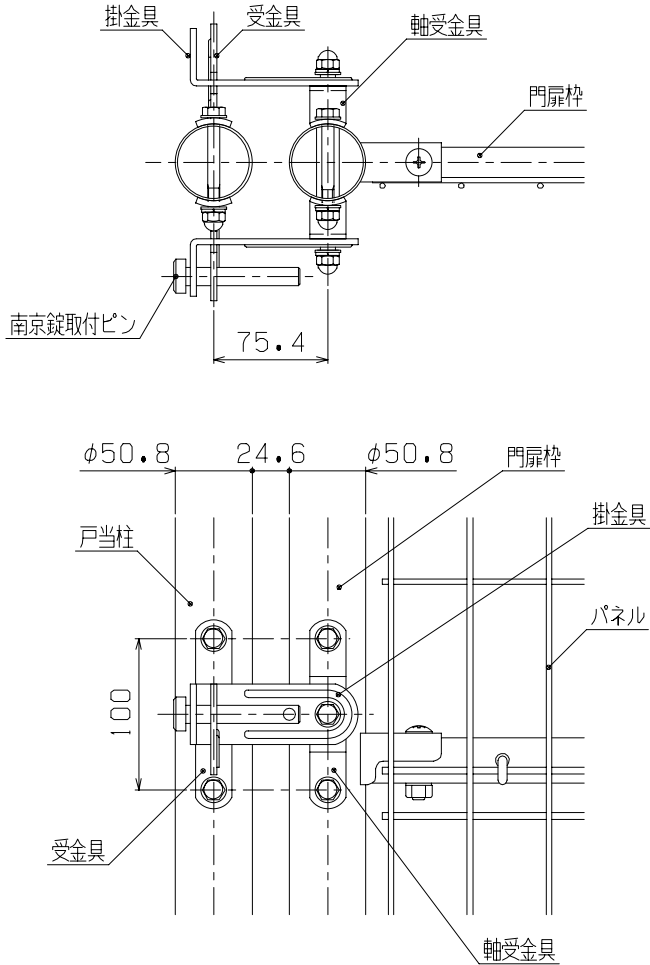
A部詳細図 (1/5)
