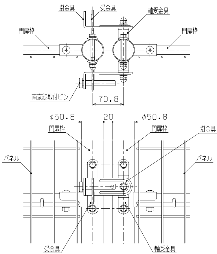
A部詳細図 (1/5)
