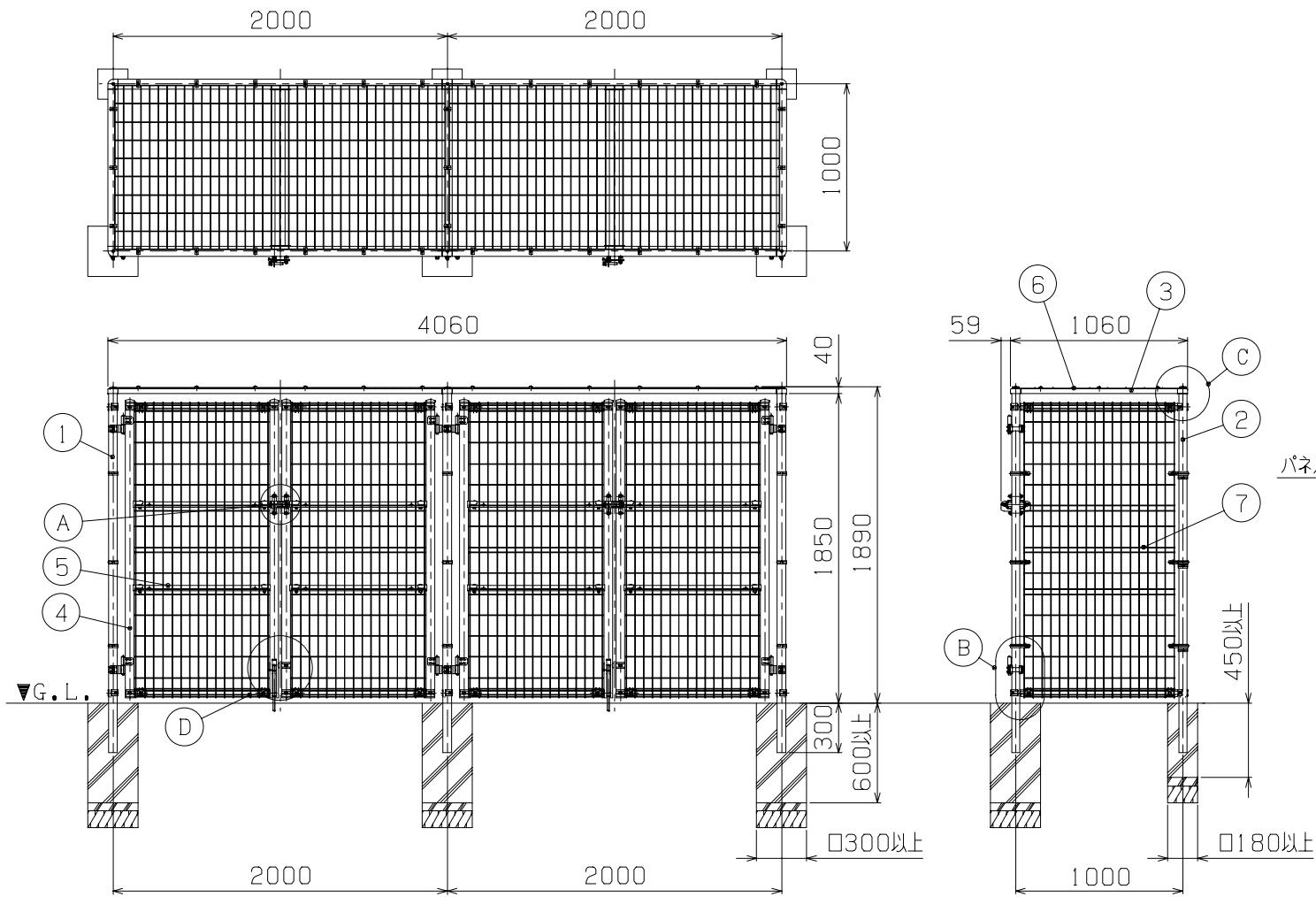
据 付 図 (1/40)
