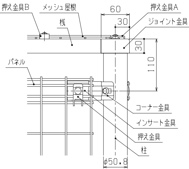
C部詳細図 (1/5)
