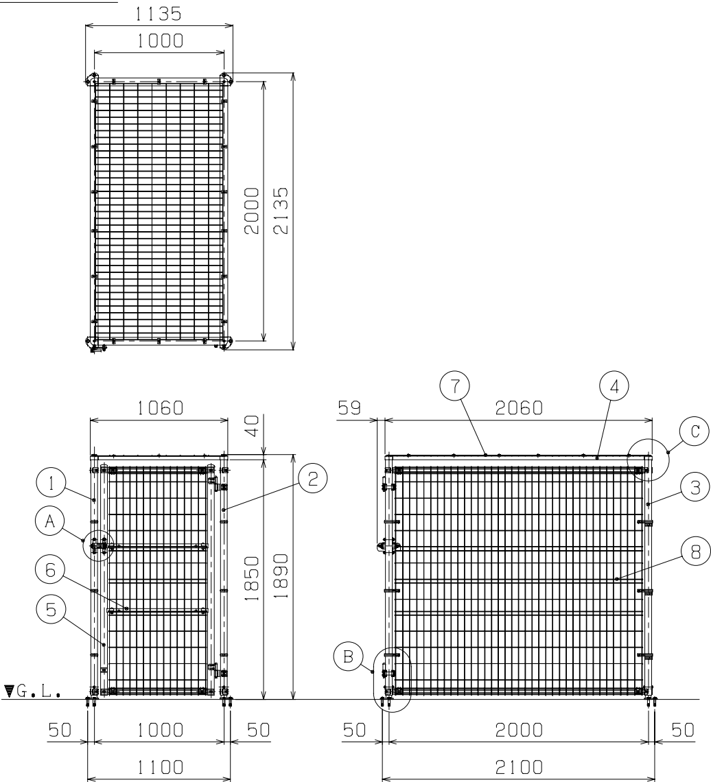
据付図 (1/40)
