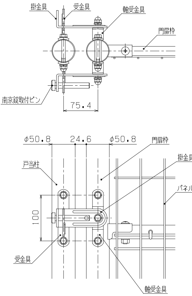
A部詳細図 (1/5)
