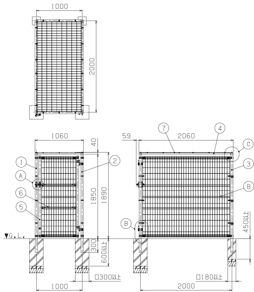
据 付 図 (1/40)
