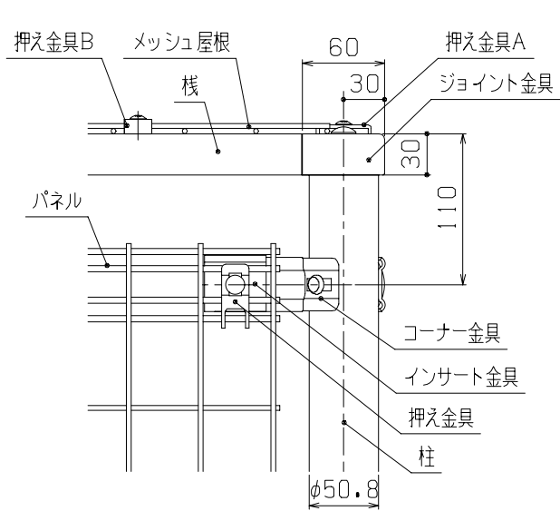
C部詳細図 (1/5)
