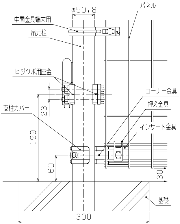
B部詳細図 (1/5)
