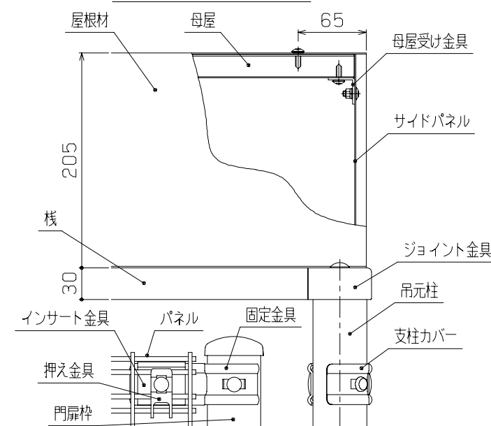
D部詳細図 (1/5)
