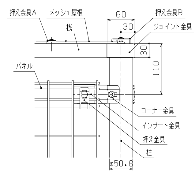
C部詳細図 (1/5)
