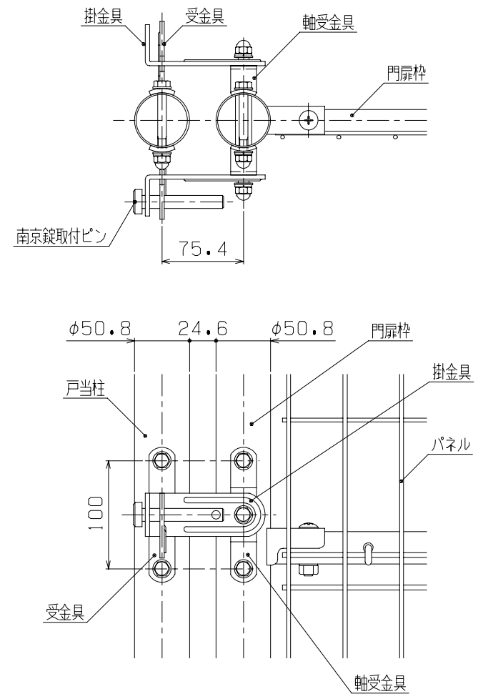
A部詳細図 (1/5)
