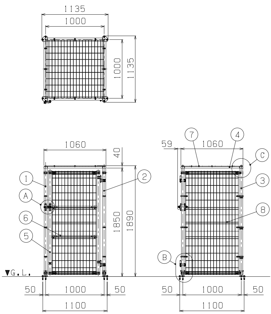
据 付 図 (1/40)
