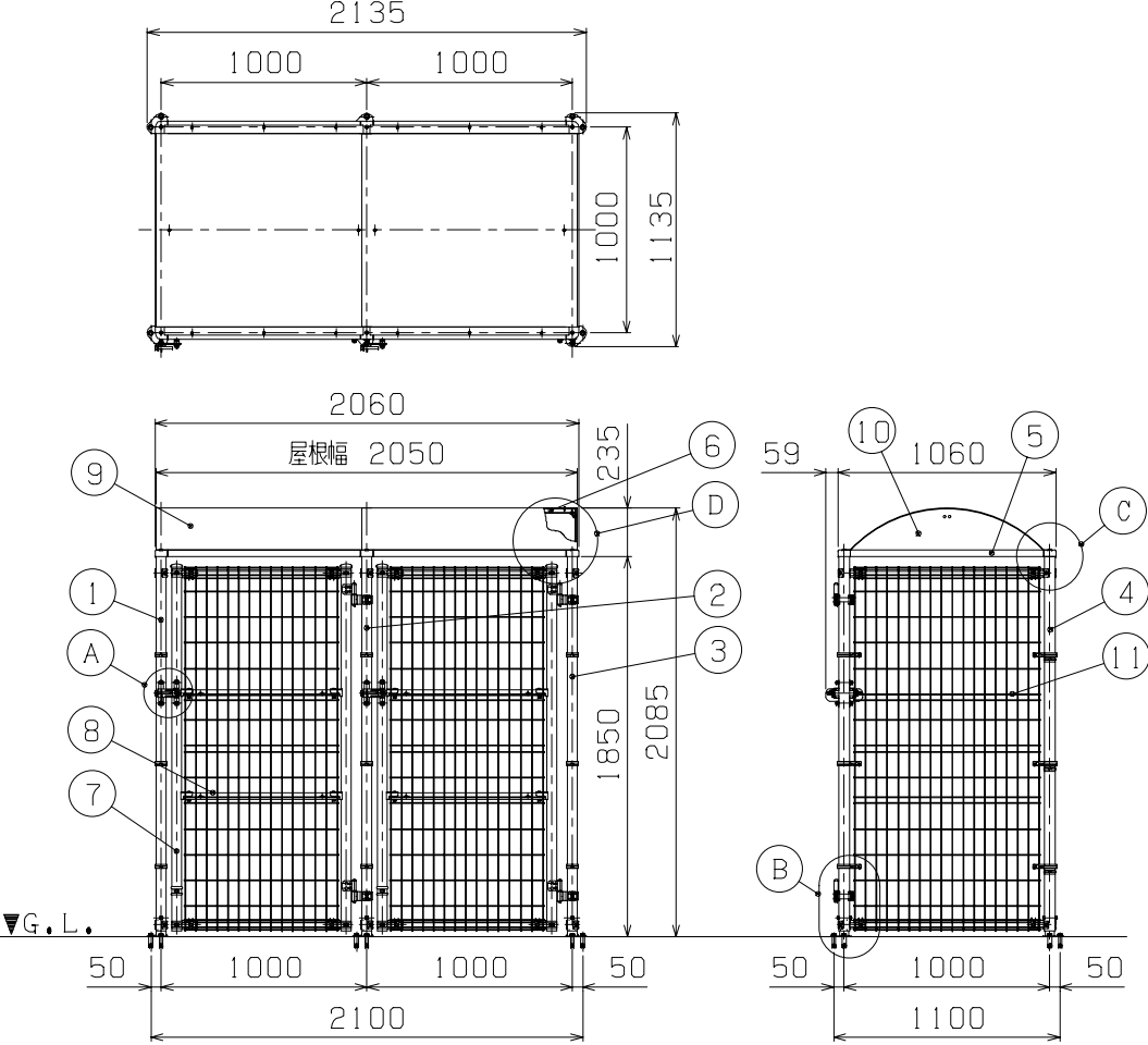
据付図 (1/40)
