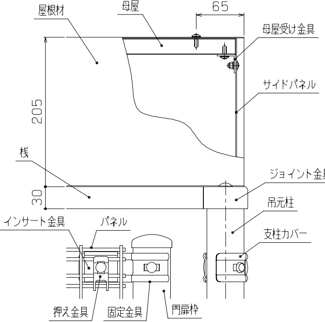
D部詳細図 (1/5)
