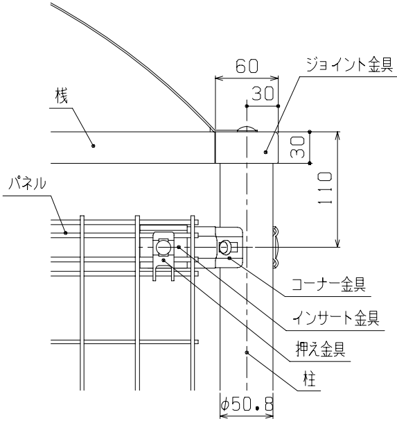
C部詳細図 (1/5)
